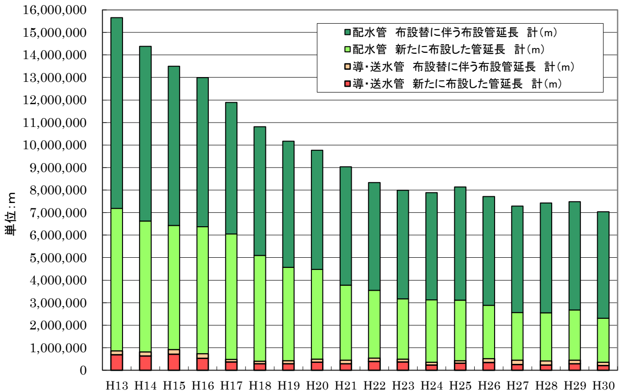
(参考図) 新設管及び布設替管の合計延長の推移(全国、上水+用供、積上げ)
