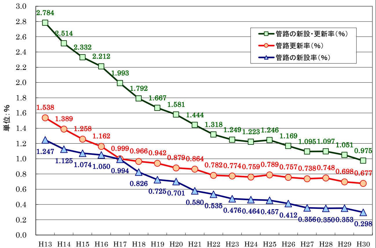
図3 管路の新設・更新率の推移(全国、上水+用供)
