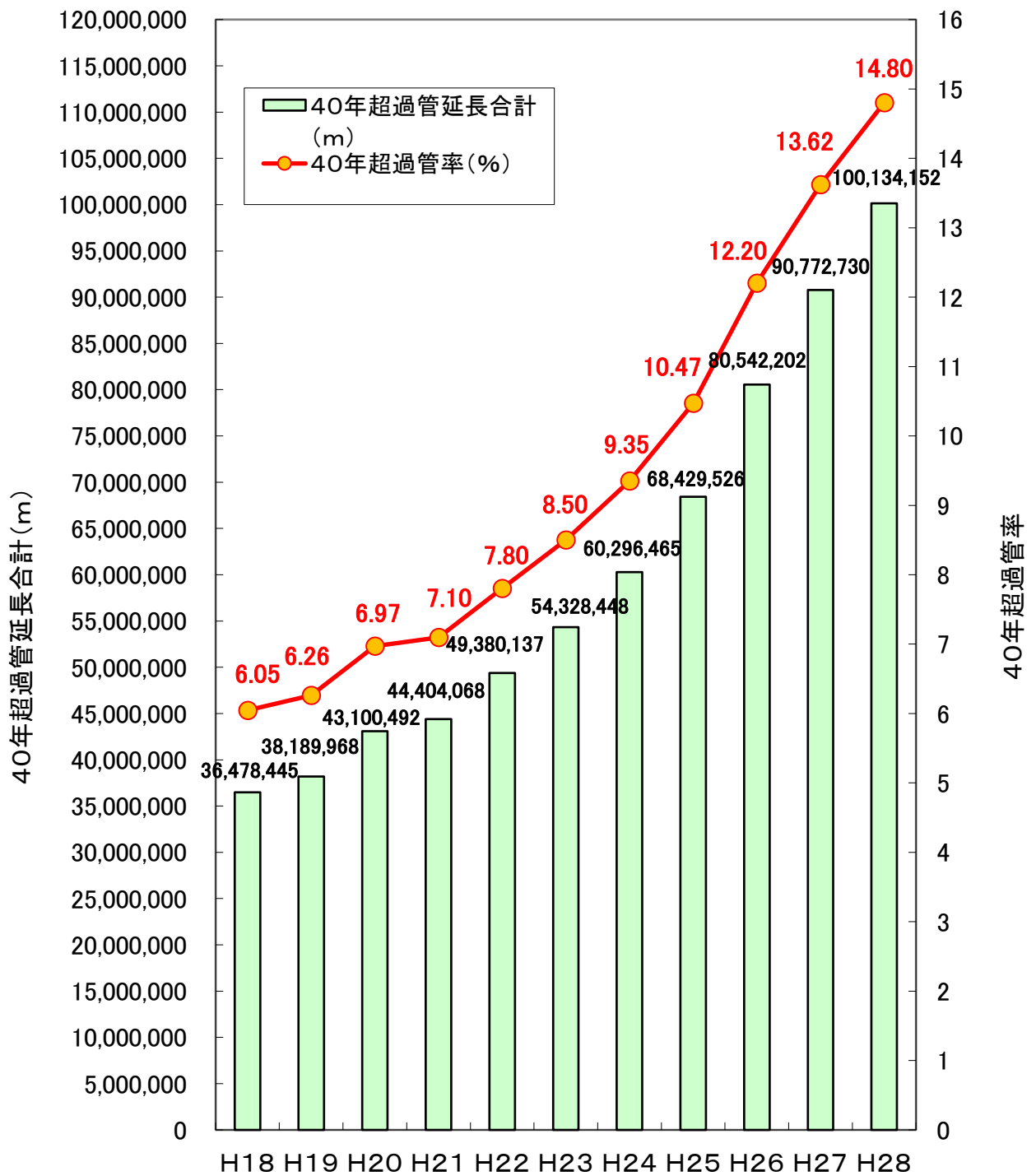
図1 40年超過管率等の推移(全国、上水+用供)
