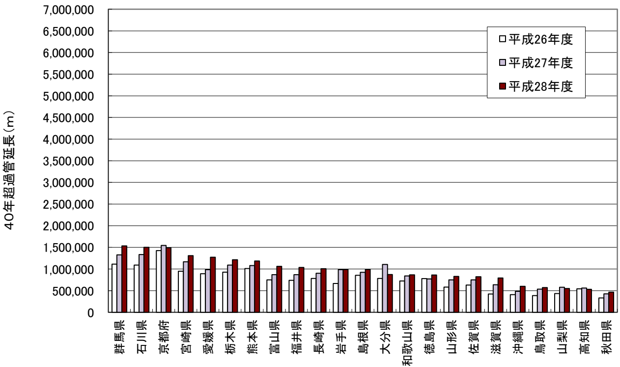
図2-2 都道府県別にみた40年超過管延長の推移(H26~H28) (平成28年度における40年超過管延長が長い順) - その2 -
