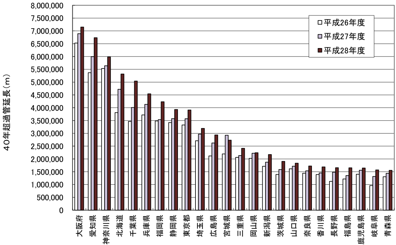
図2-1 都道府県別にみた40年超過管延長の推移(H26~H28) (平成28年度における40年超過管延長が長い順) - その1 -
