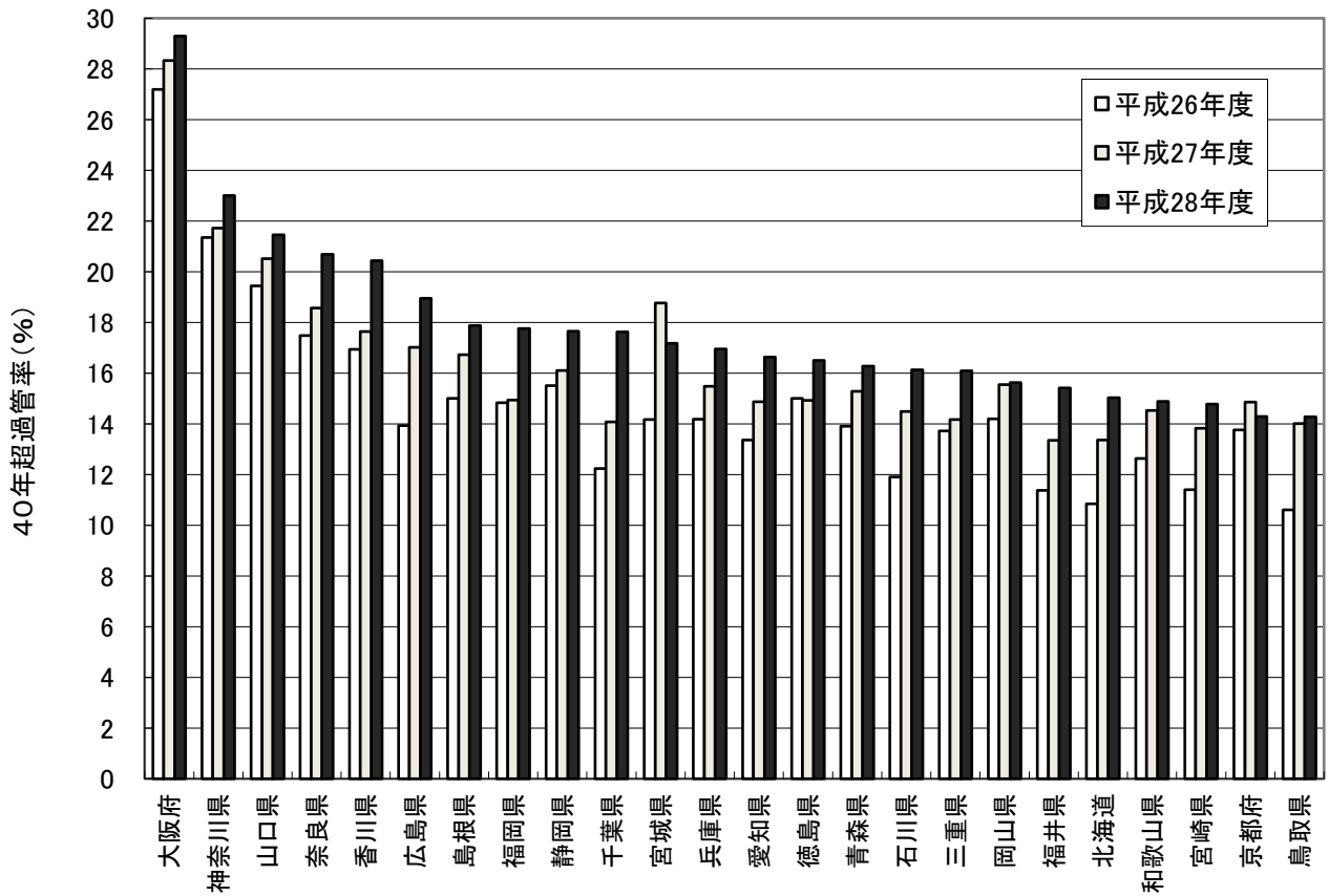
図3-1 都道府県別にみた40年超過管率の推移(平成26~28年度) -平成28年度超過管率の高い順-(その1)
