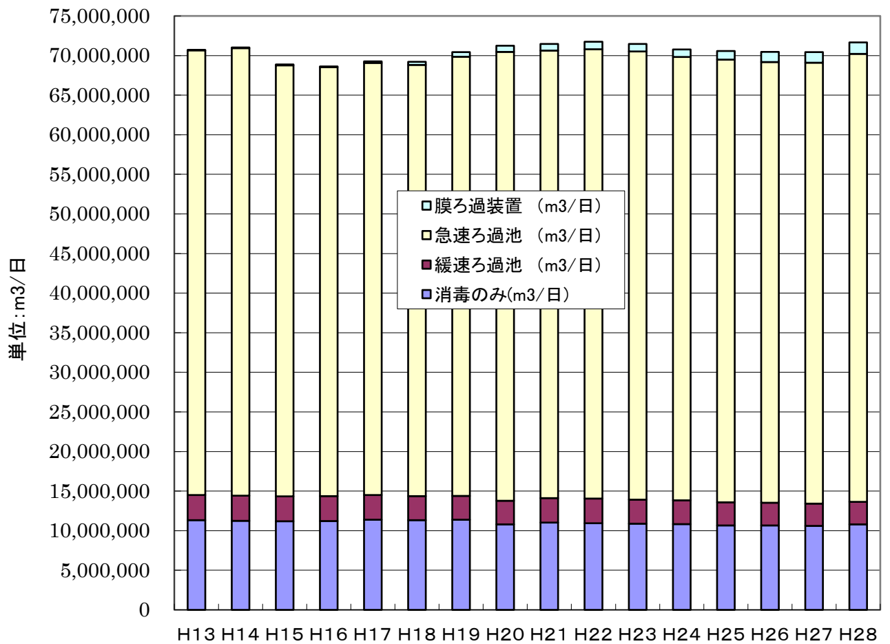
図2-1 浄水方法別計画浄水量の推移(用供+上水)ー積み上げー JWRC
