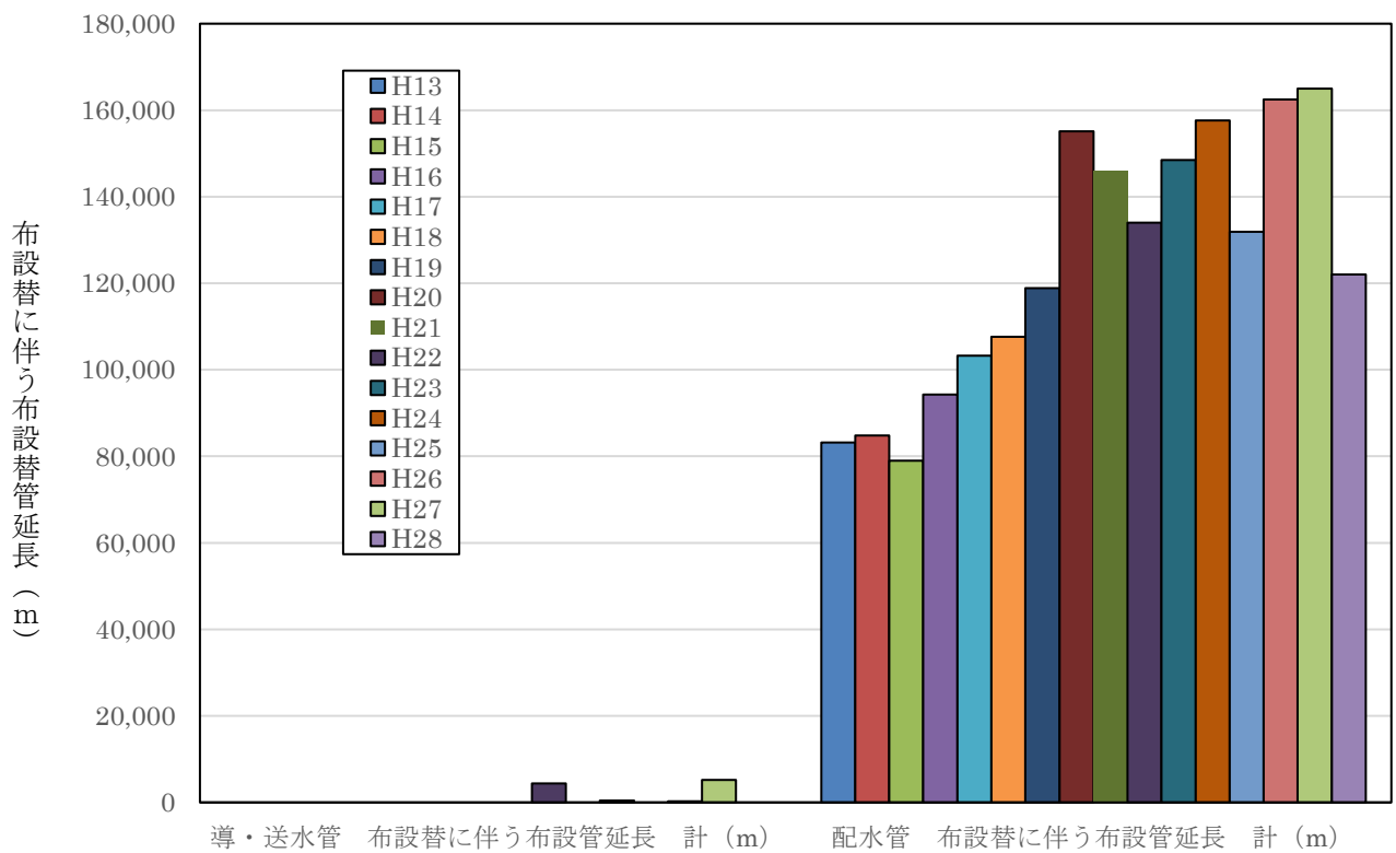
図2-5-2 導・送水管及び配水管別にみた布設替に伴う布設管延長の推移 (横浜市)
