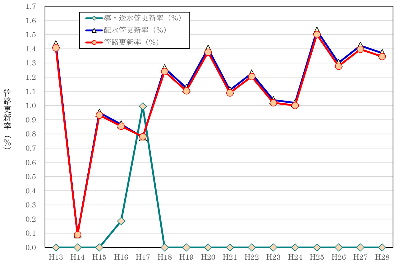
図2-2-1 導・送水管及び配水管別にみた管路更新率の推移 (大阪市)
