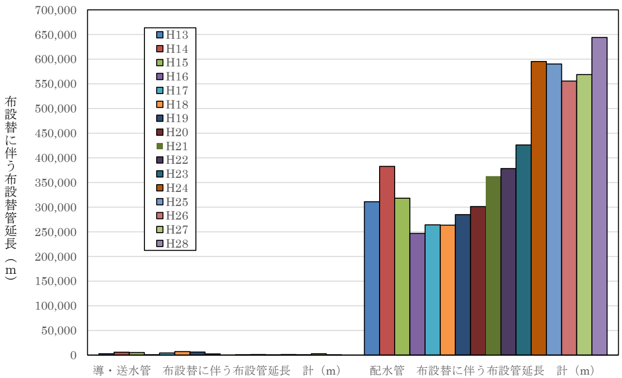
図2-1-2 導・送水管及び配水管別にみた布設替に伴う布設管延長の推移 (東京都)
