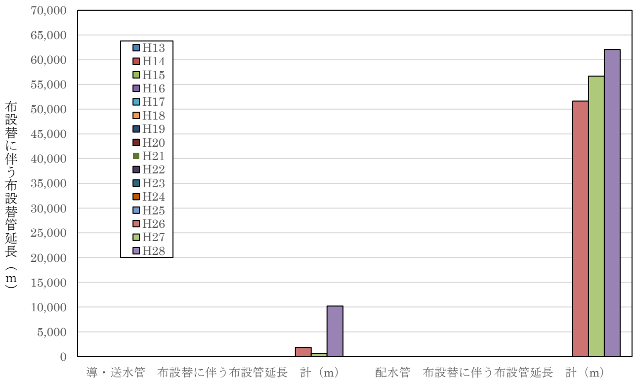
図2-3-2 導・送水管及び配水管別にみた布設替に伴う布設管延長の推移 (神奈川県)
