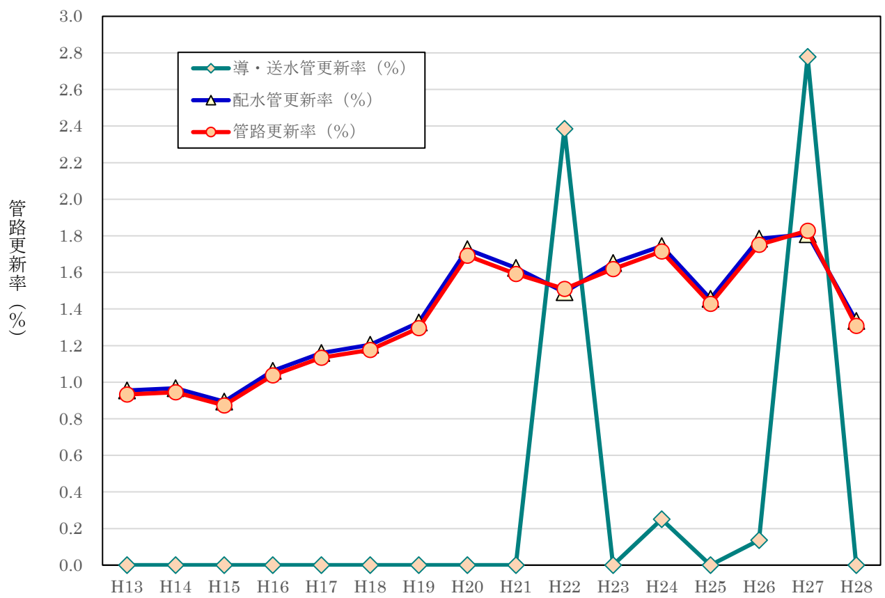
図2-5-1 導・送水管及び配水管別にみた管路更新率の推移 (横浜市)
