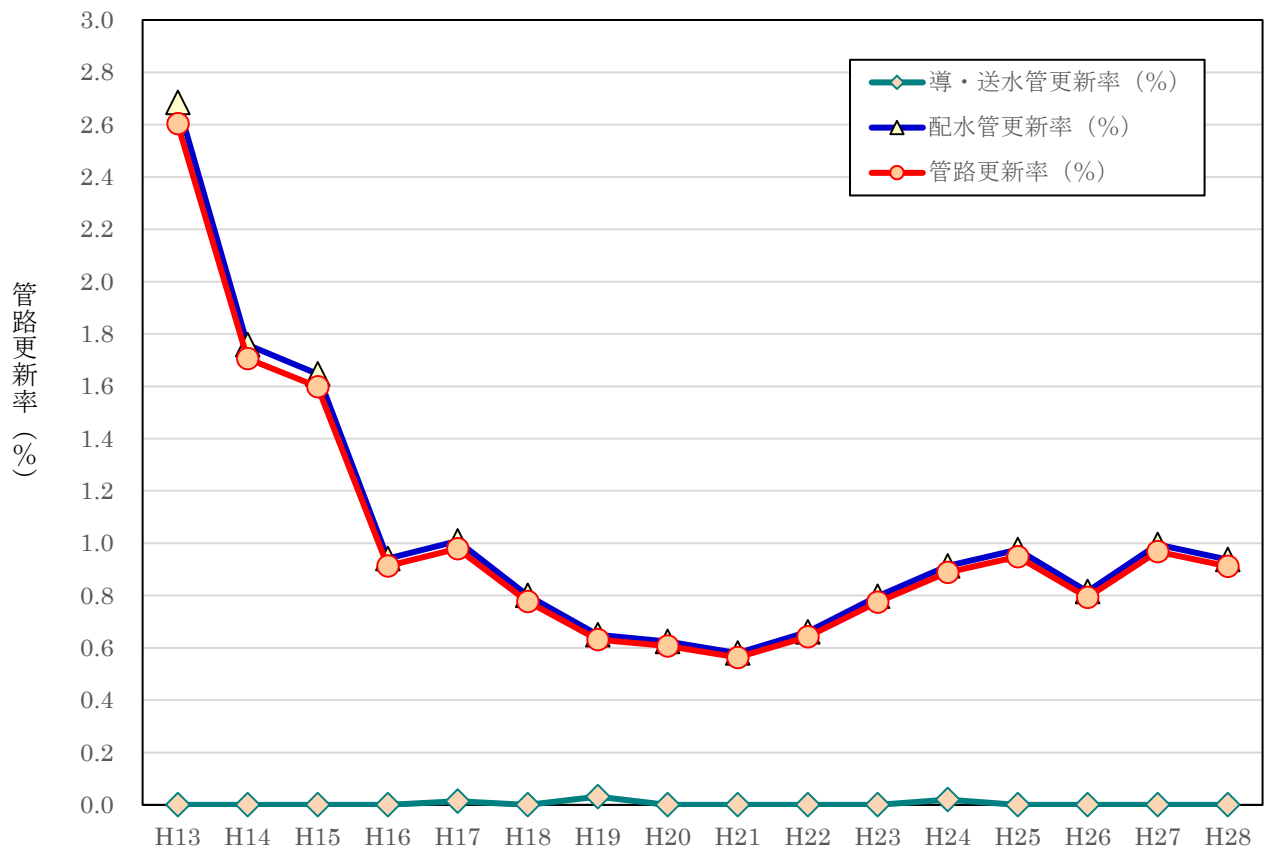
図2-4-1 導・送水管及び配水管別にみた管路更新率の推移 (千葉県)
