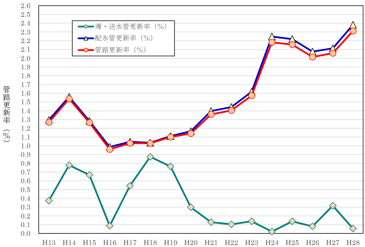
図2-1-1 導・送水管及び配水管別にみた管路更新率の推移 (東京都)
