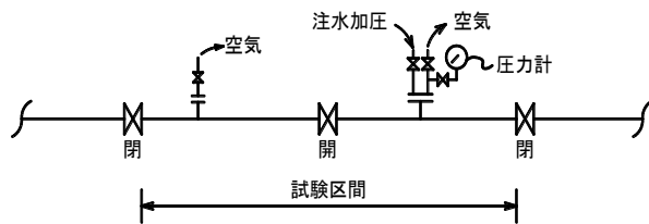
図1 管路水圧試験例
