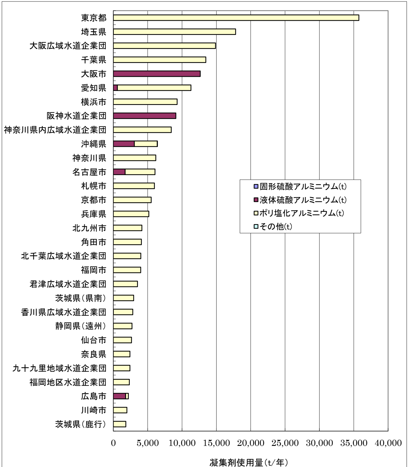
図2 凝集剤の種類別使用状況(凝集剤使用量の多い上位30事業体)
