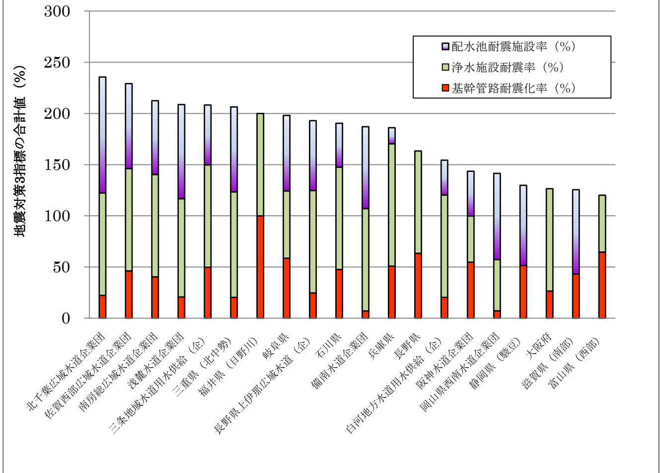
図4 平成18年度における地震対策3指標の高い水道用水供給20事業者 (平成18年度水道統計に基づく試算結果)
