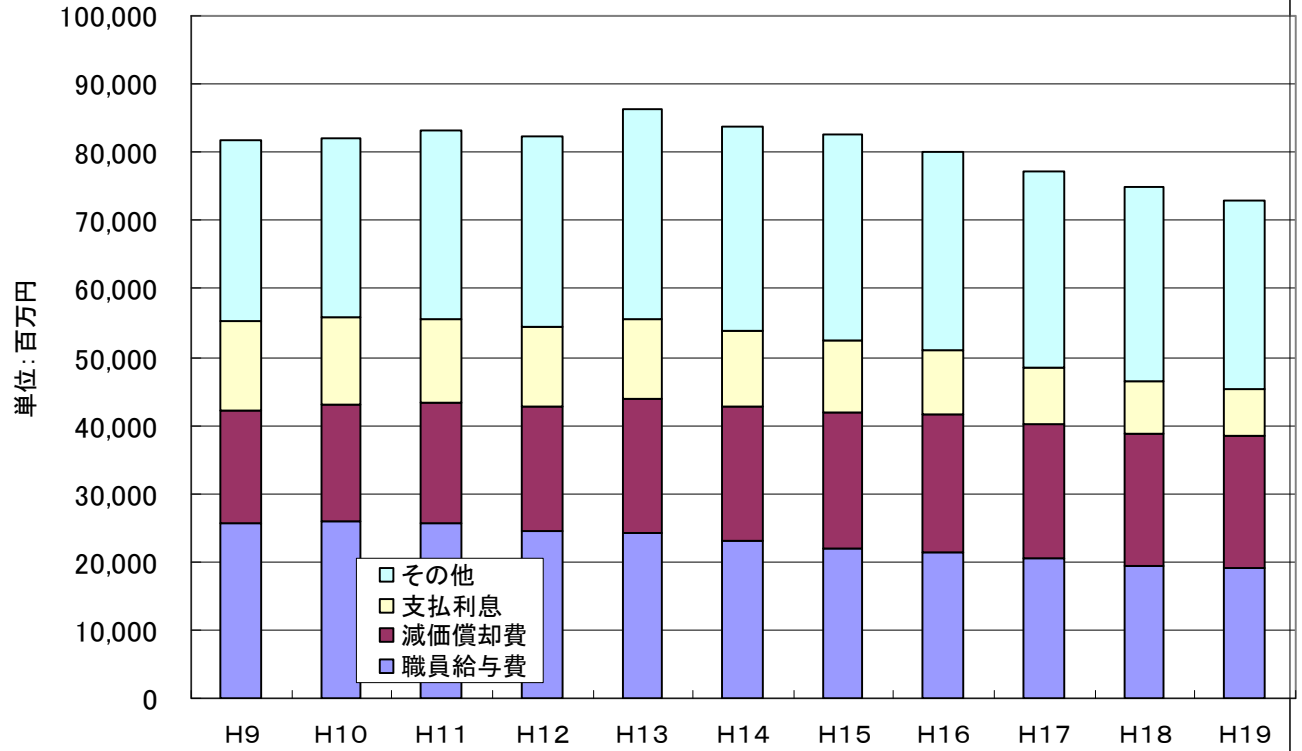
図6-4-1 電気事業における経常費用の内訳
