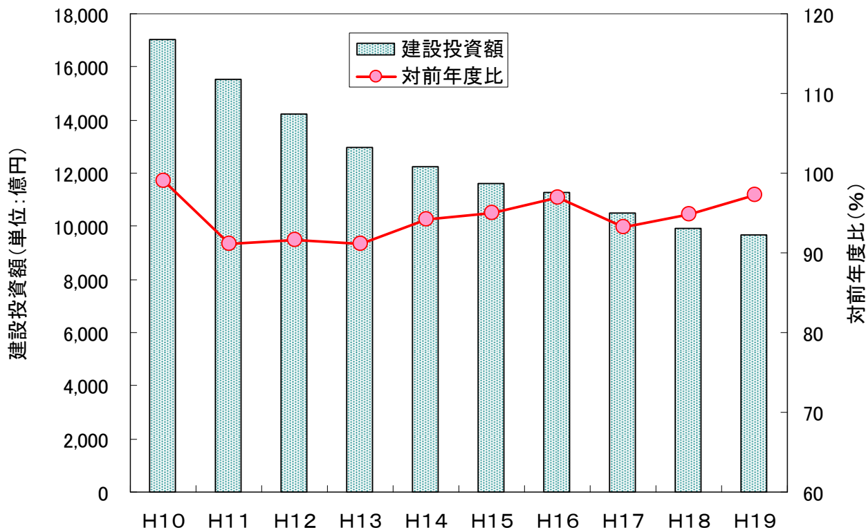
参考図1 建設投資額と対前年度比—上水道事業—
