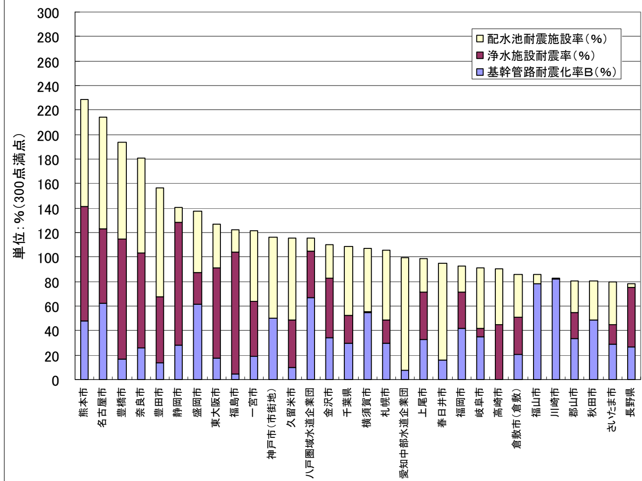
図4 平成19年度地震対策3指標合計 (計画給水人口20万人以上の上水道事業、3指標合計値の高い30事業)
