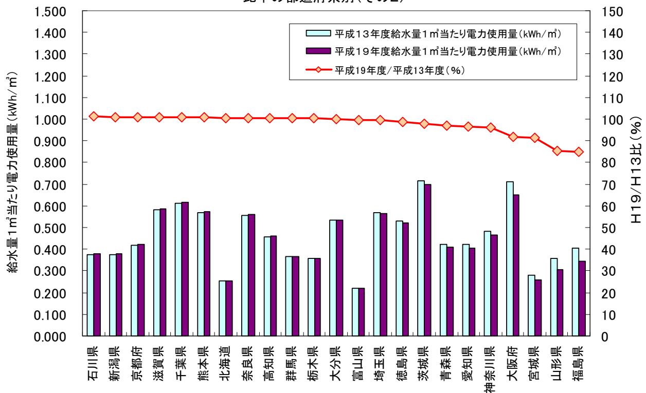
図5-2 給水量1m 3 当たり電力使用量(H19/H13比) —比率の都道府県別(その2)—
