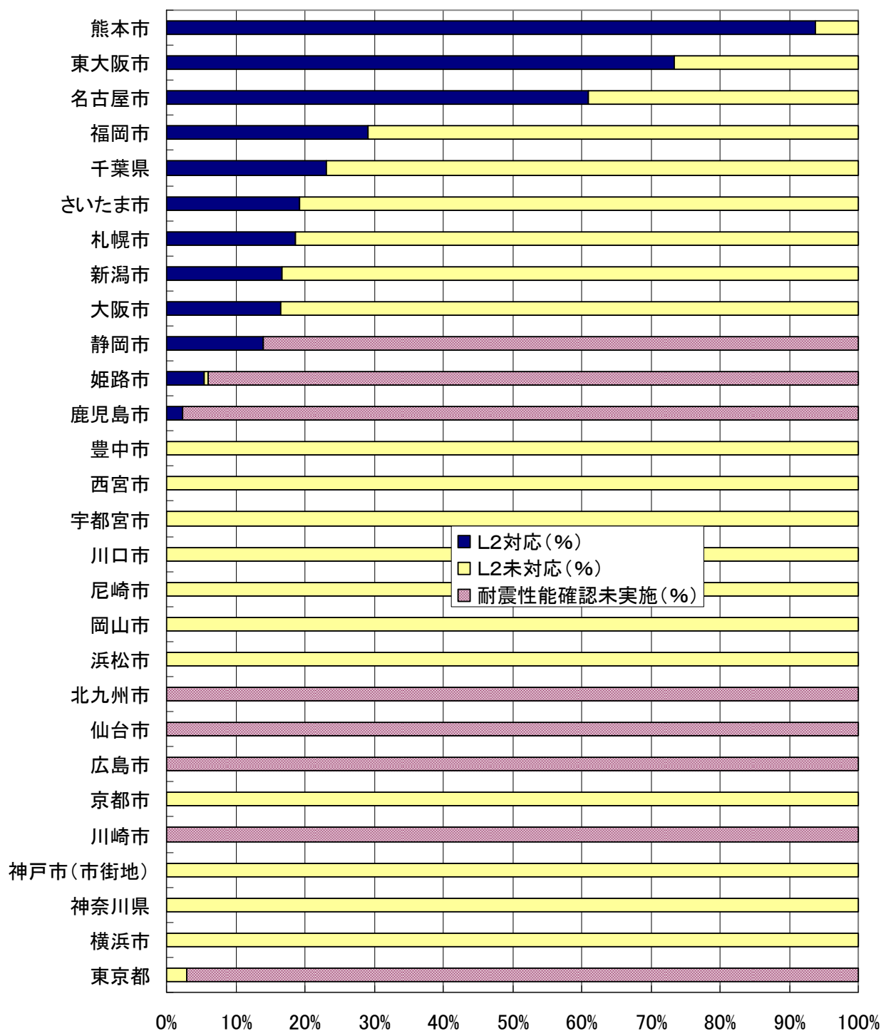
図 現在給水人口50万人以上の上水道29事業体の 浄水施設耐震施設率等(平成20年度)
