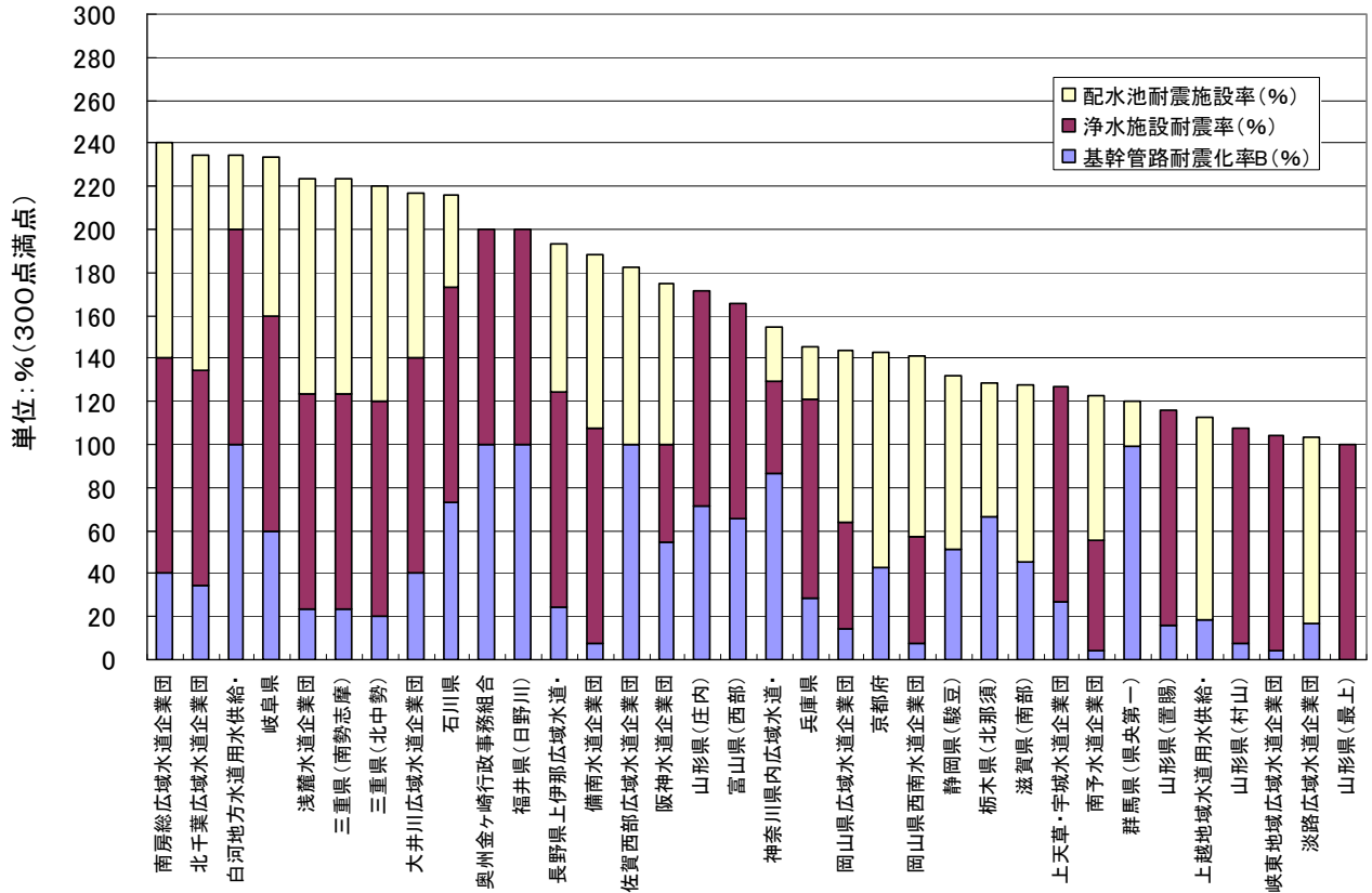
図3-1 水道用水供給101事業の地震対策3指標合計値(平成20年度)―その1―
