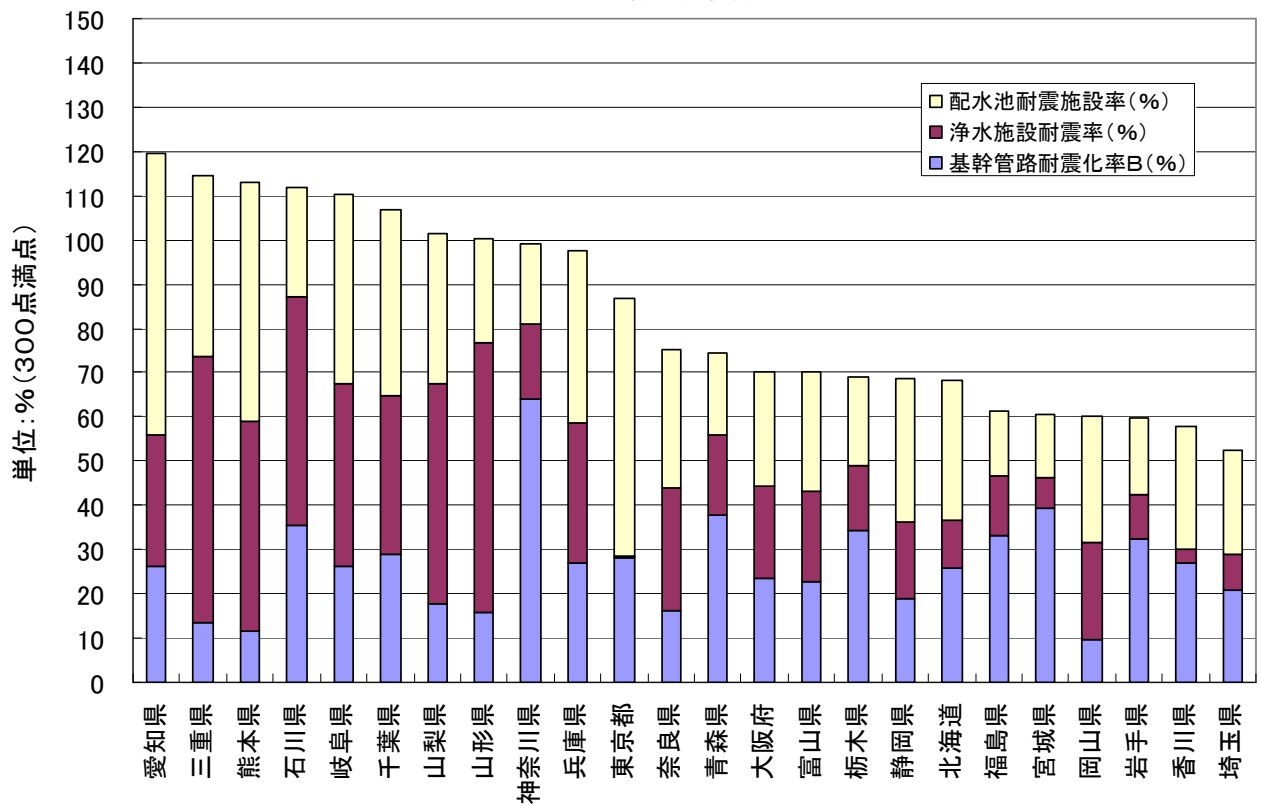
図2-1 都道府県別にみた地震対策3指標合計値(平成20年度)－その1－ (値の大きい都道府県順)
