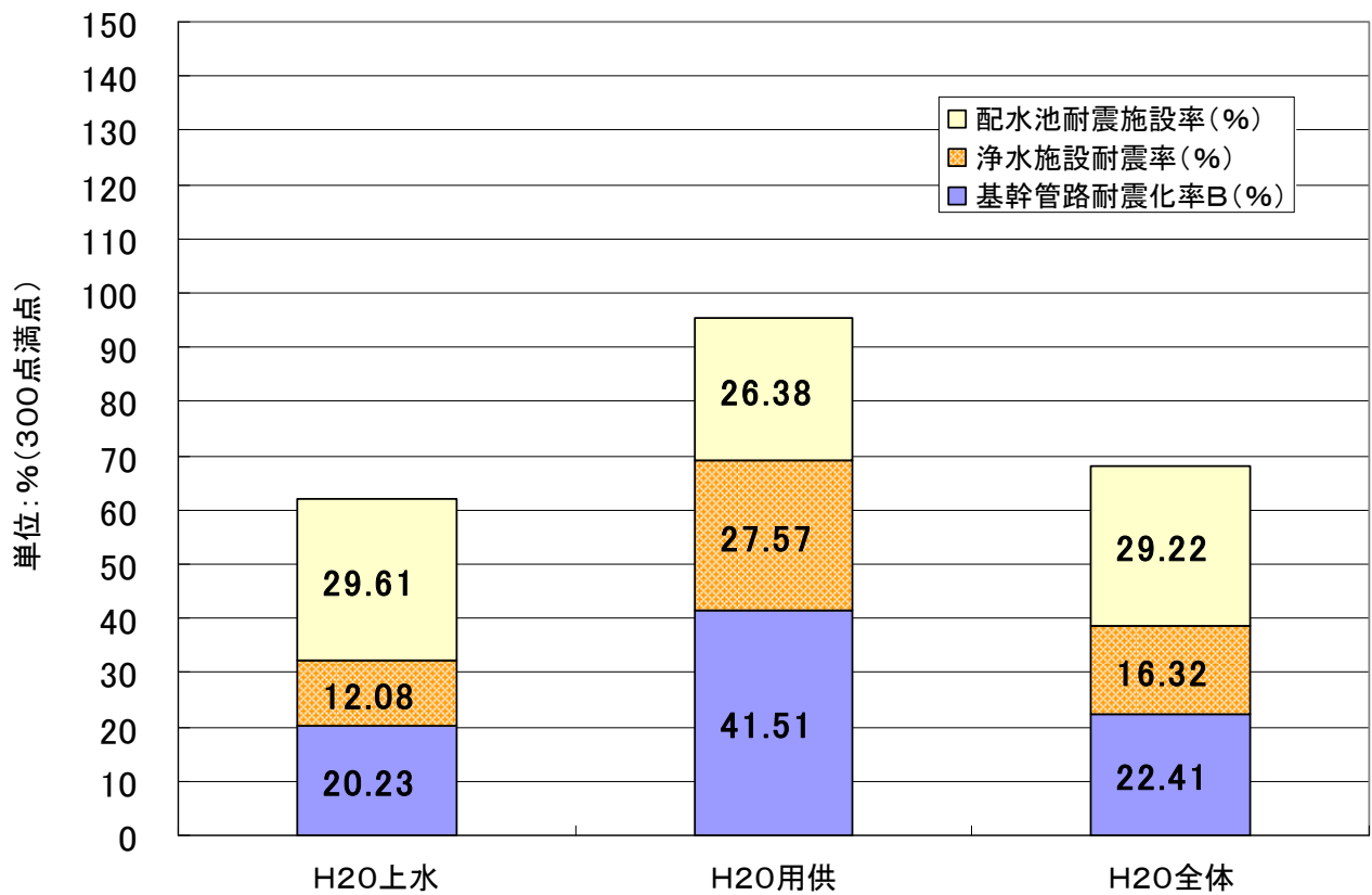
図1-1 平成20年度における地震対策3指標の合計値(全国、上水・用供)
