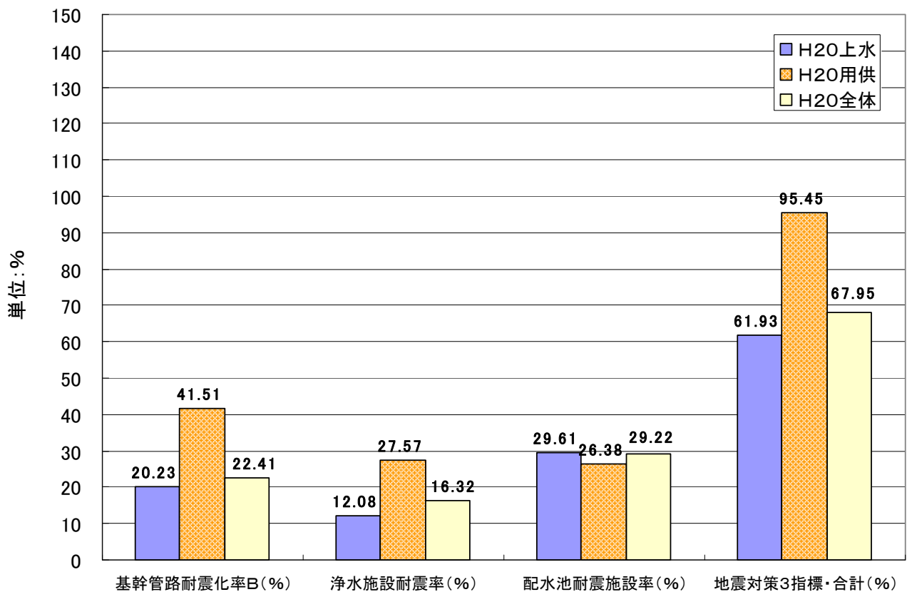
図1-2 平成20年度における地震対策3指標の合計値(全国、上水・用供)
