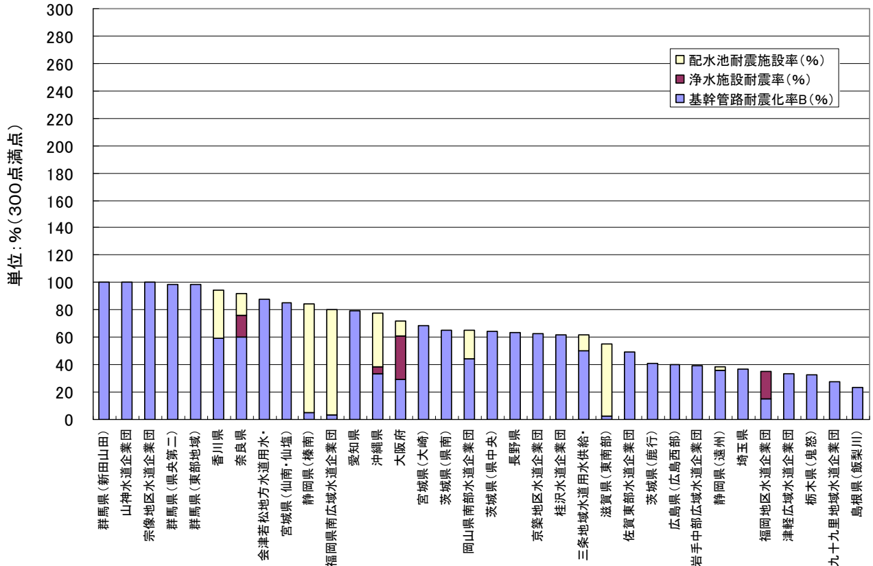
図3-2 水道用水供給101事業の地震対策3指標合計値(平成20年度)―その2―
