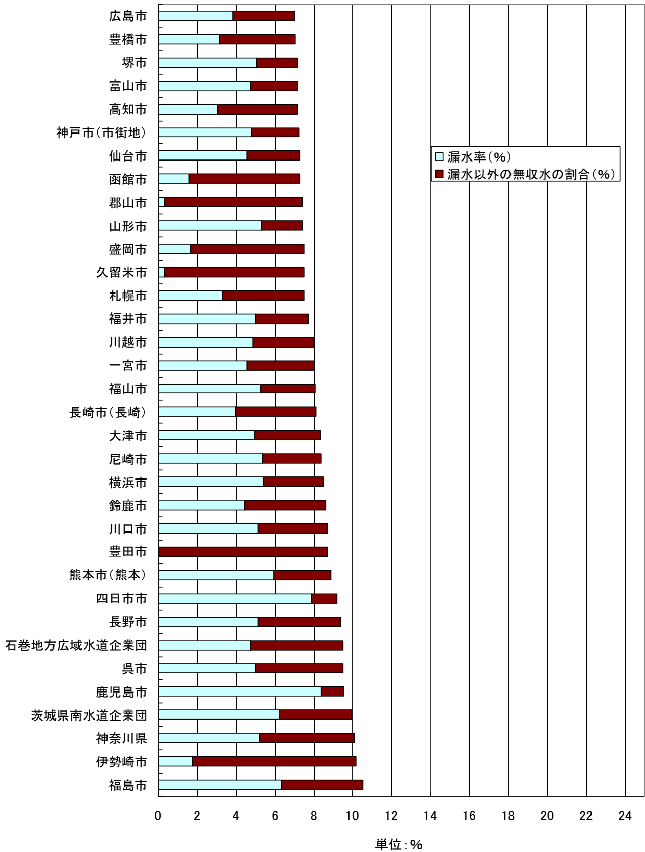
図3-2 現在給水人口20万人以上の上水道100事業における無収水率(平成21年度) -その2-
