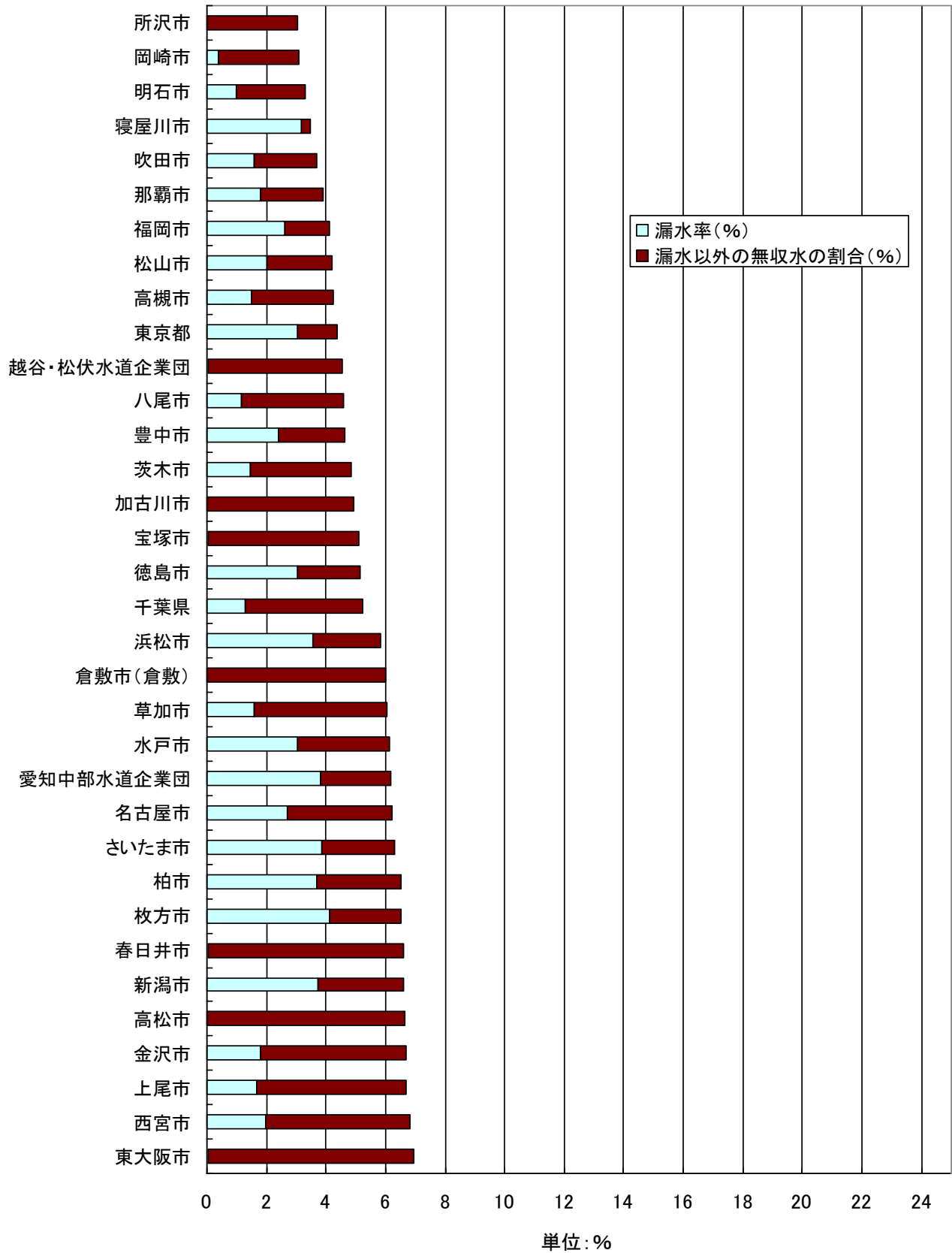
図3-1 現在給水人口20万人以上の上水道100事業における無収水率(平成21年度) -その1-
