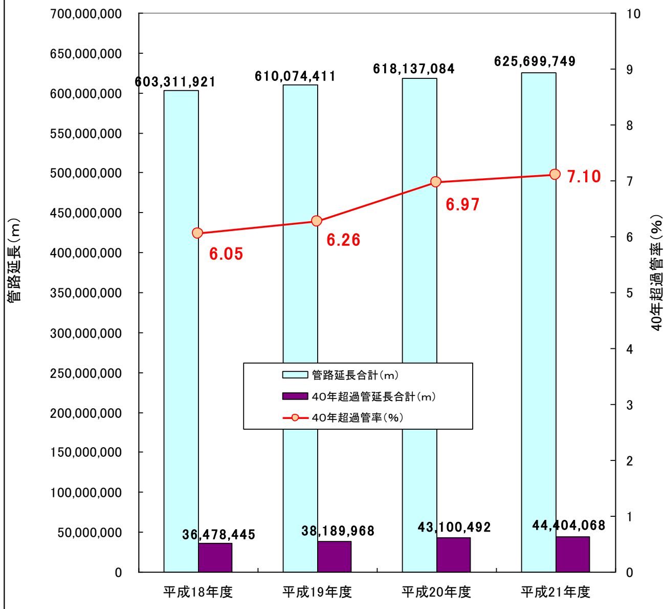
図1 40年超過管率等の推移(全国、上水+用供)
