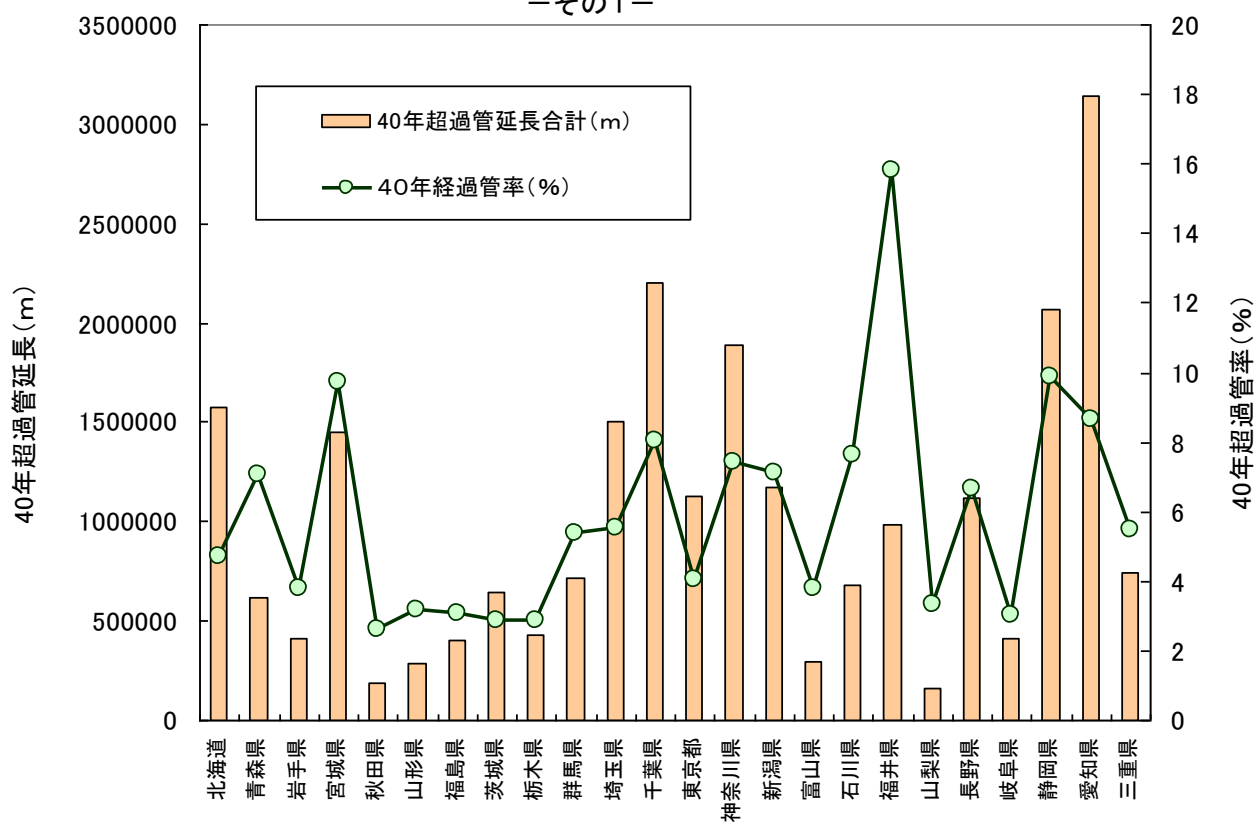
図2-1 都道府県別にみた40年超過管延長及び40年超過管率(平成21年度) -その1-
