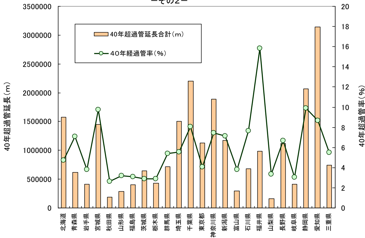
図2-2 都道府県別にみた40年超過管延長及び40年超過管率(平成21年度) -その2-
