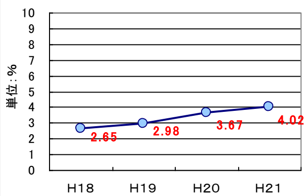
図3-13 40年超過管率の推移(東京都)
