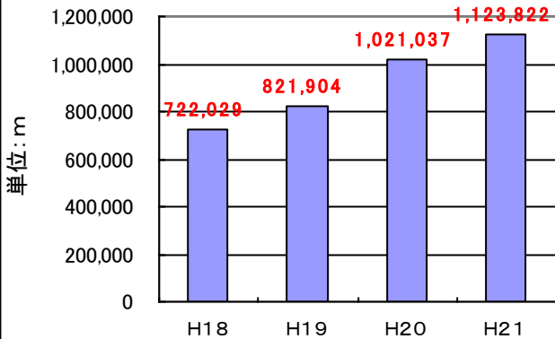
図2-13 40年超過管延長の推移(東京都)
