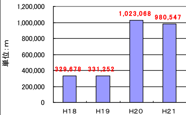
図2-18 40年超過管延長の推移(福井県)
