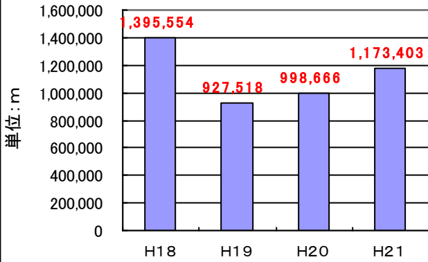
図2-15 40年超過延長の推移(新潟県)
