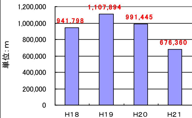
図2-17 40年超過管延長の推移(石川県)
