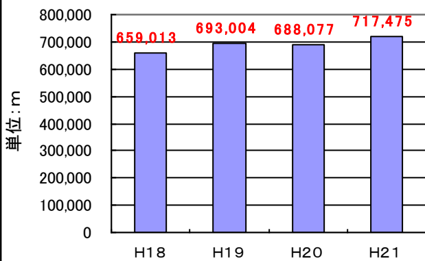
図2-10 40年超過管延長の推移(群馬県)
