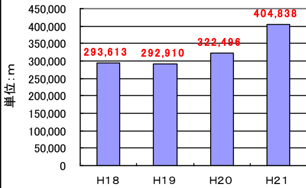
図2-7 40年超過管延長の推移(福島県)
