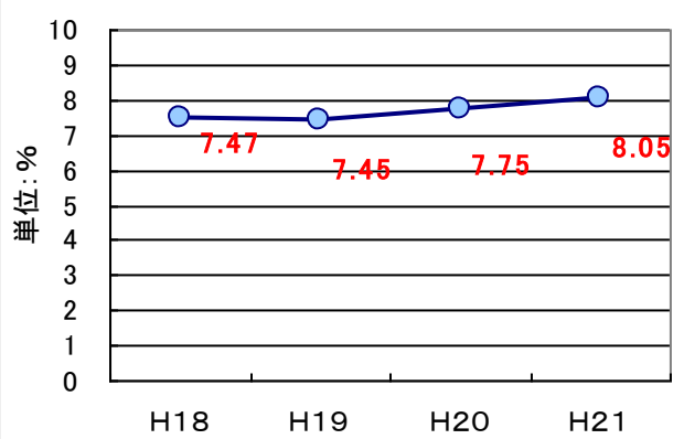
図3-12 40年超過管率の推移(千葉県)
