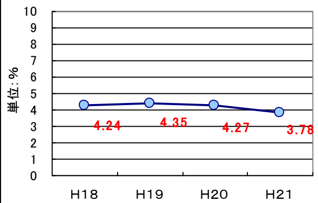
図3-3 40年超過管率の推移(岩手県)
