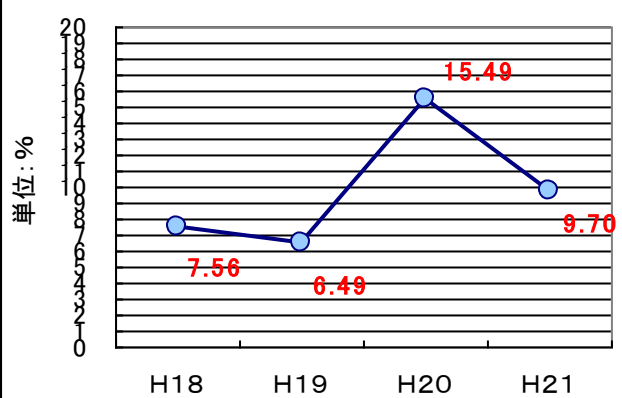
図3-4 40年超過管率の推移(宮城県)
