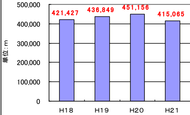
図2-3 40年超過管延長の推移(岩手県)
