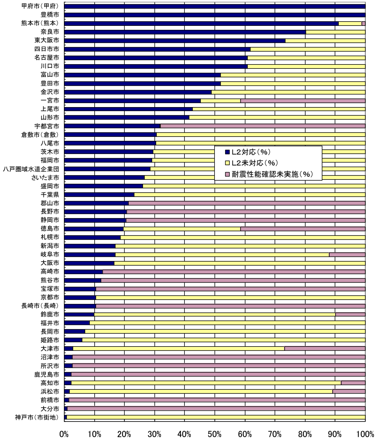
参考図1 現在給水人口20万人以上の上水道100事業者の 浄水施設耐震施設率等(平成21年度)－その1－
