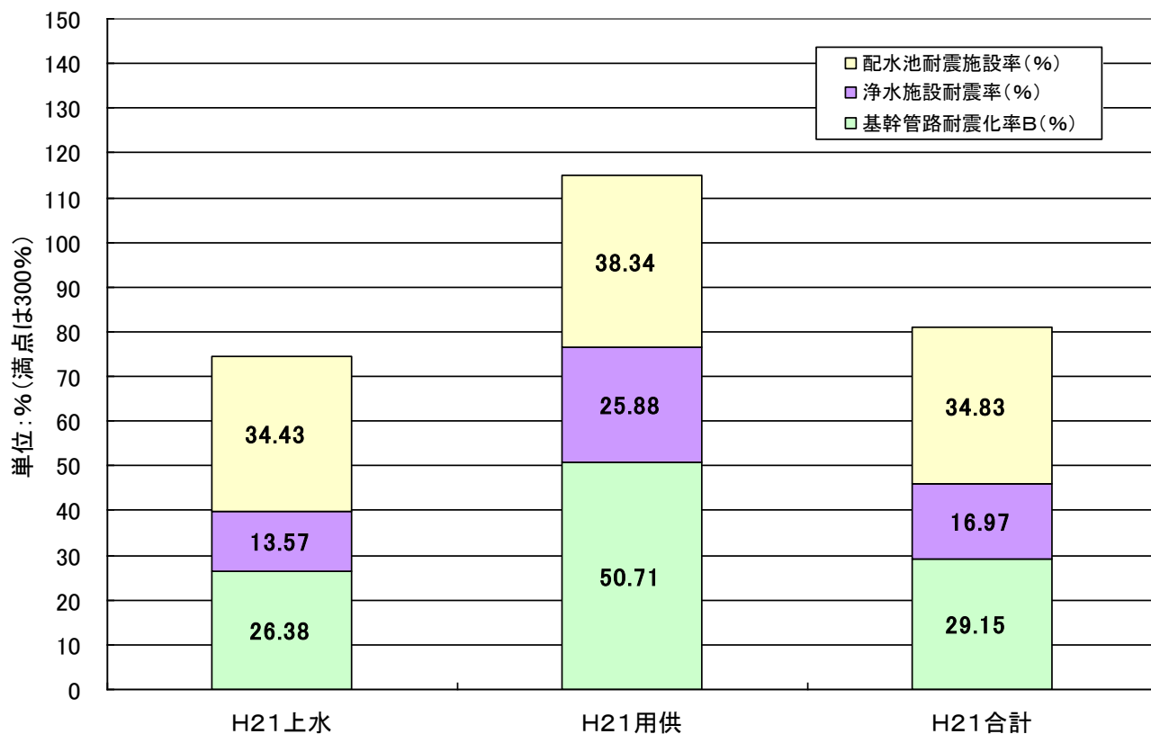
図1-1 平成21年度における地震対策3指標の合計値(全国、上水+用水)
