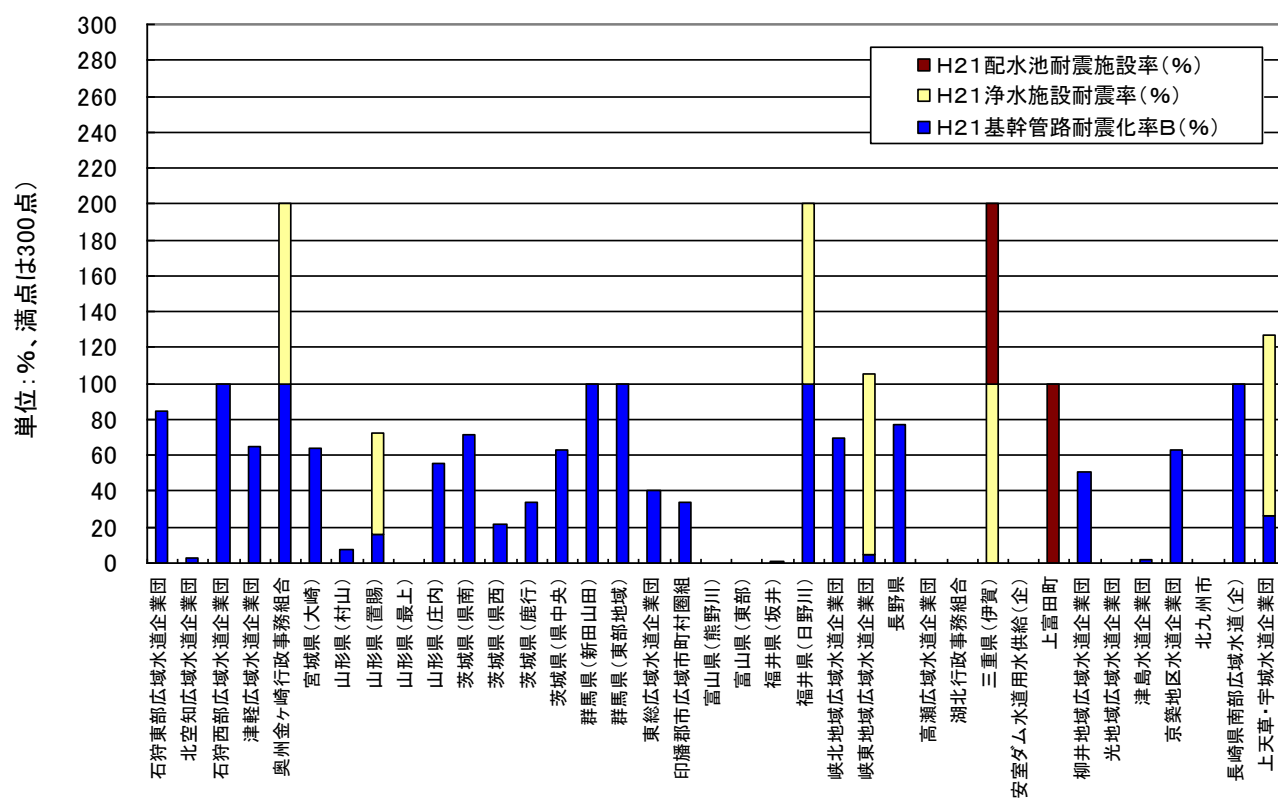
(参考図) 水道用水供給101事業の地震対策3指標合計値(平成21年度) (「#DIV/0!」が含まれる事業体)
