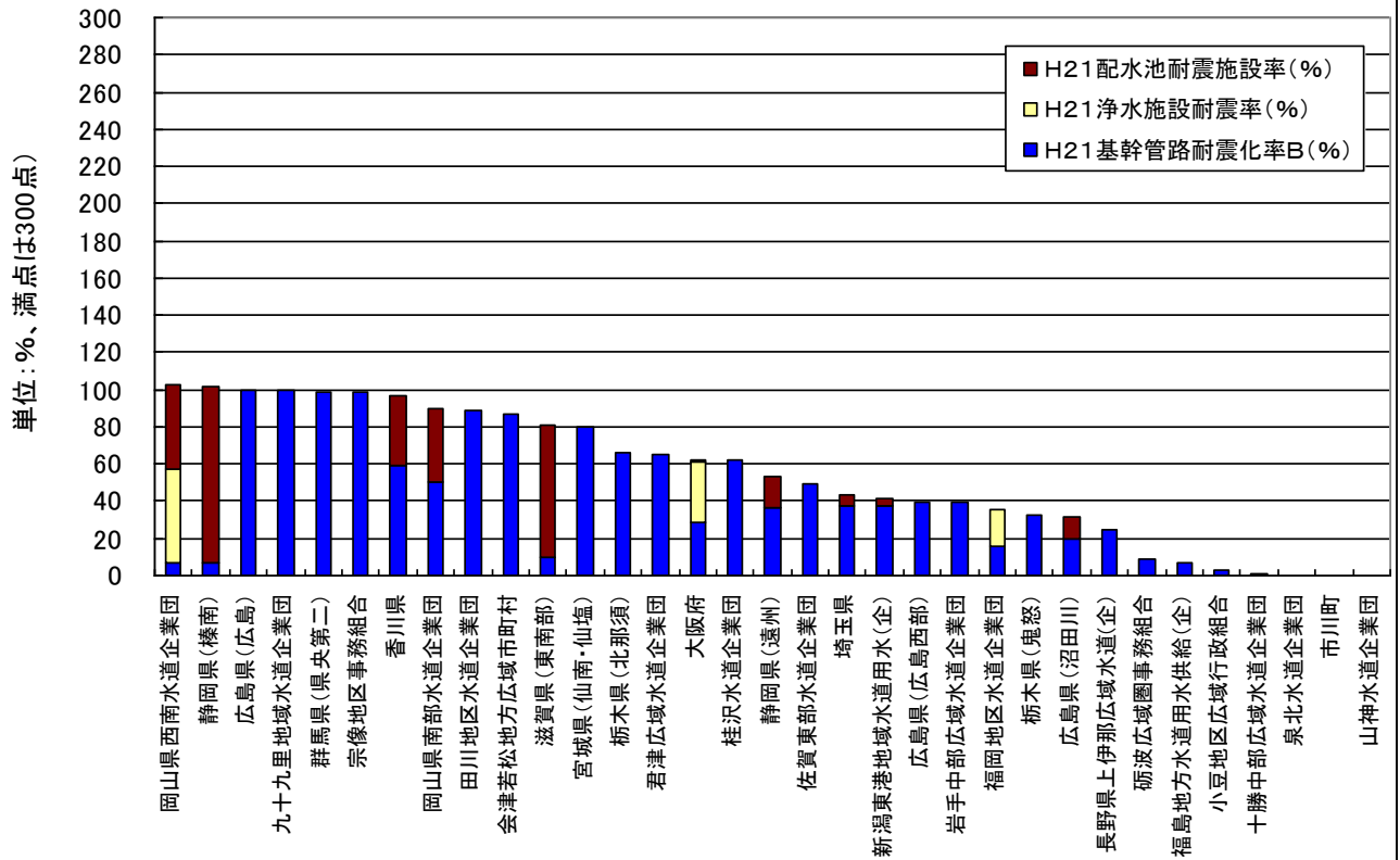
図3-2 水道用水供給101事業の地震対策3指標合計値(平成21年度) (率の高い事業体順) - その2 -
