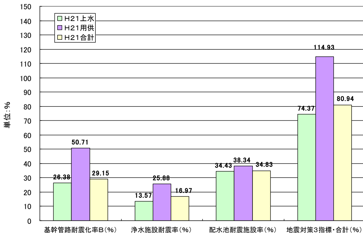
図1-2 平成21年度における地震対策3指標の合計値(全国、上水+用水)
