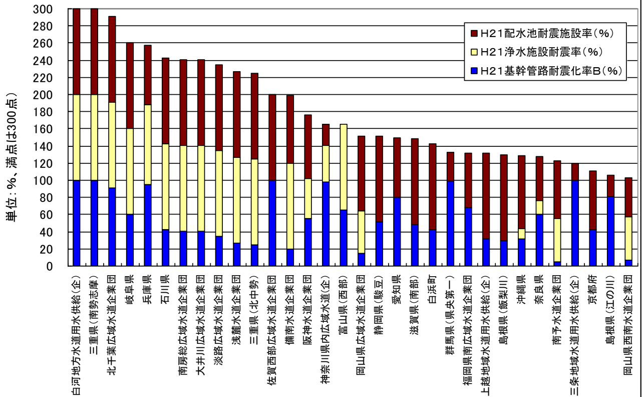
図3-1 水道用水供給101事業の地震対策3指標合計値(平成21年度) (率の高い事業体順) - その1 -
