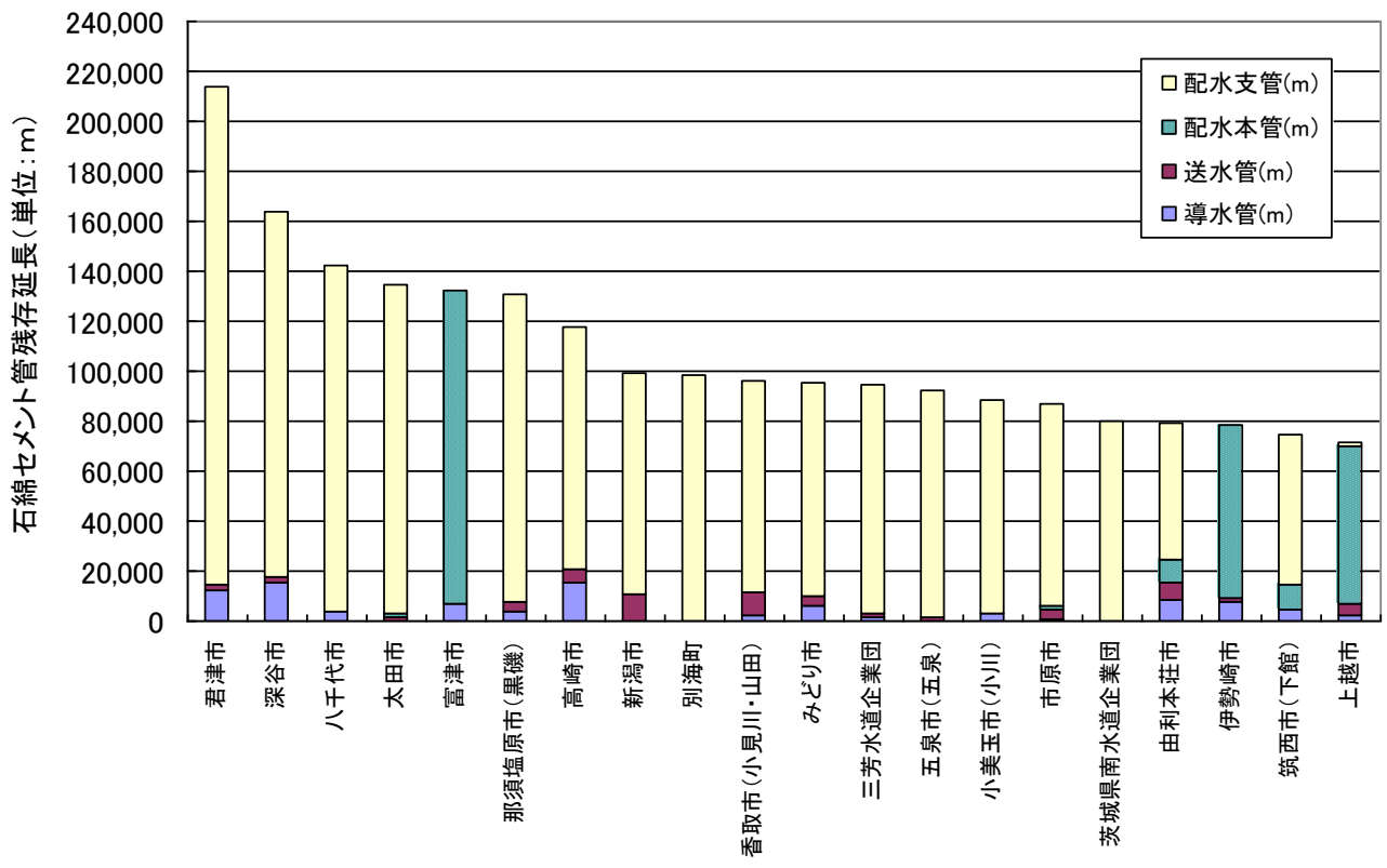
参考図3 石綿セメント管残存延長の多い事業体順 (平成19年度,上位20事業体)
