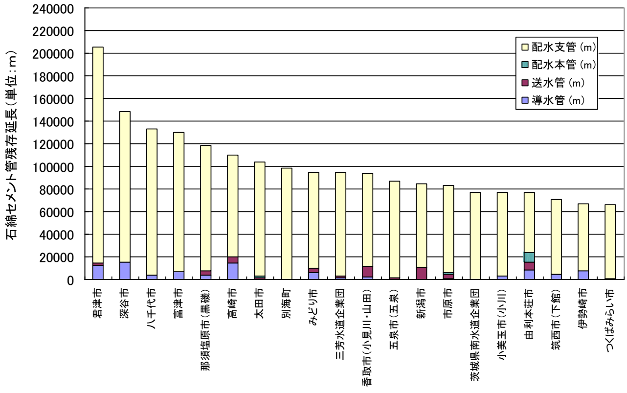
参考図2 石綿セメント管残存延長の多い事業体順 (平成20年度,上位20事業体)
