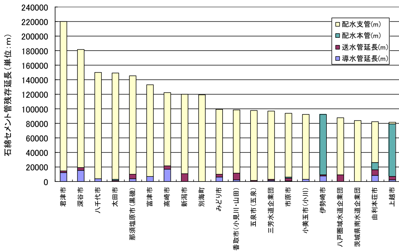
参考図4 石綿セメント管残存延長の多い事業体順 (平成18年度,上位20事業体)
