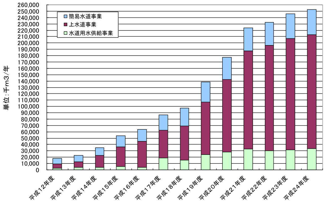
図1 膜ろ過浄水施設(MF・UF・NF・ROの合計)による年間実浄水量の推移(積上げ)
