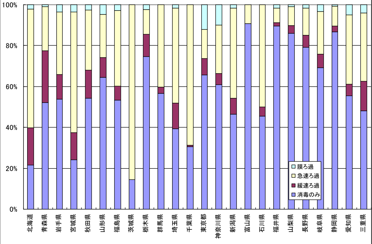
図3-3 都道府県別にみた浄水方法別浄水場数(平成24年度、その3) - 構成割合 -
