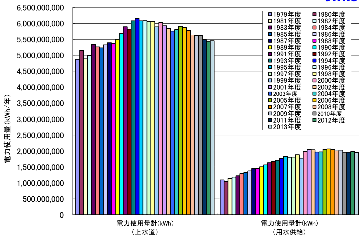
図1-2 水道施設(上水道・用水供給別)における電力使用量の推移
