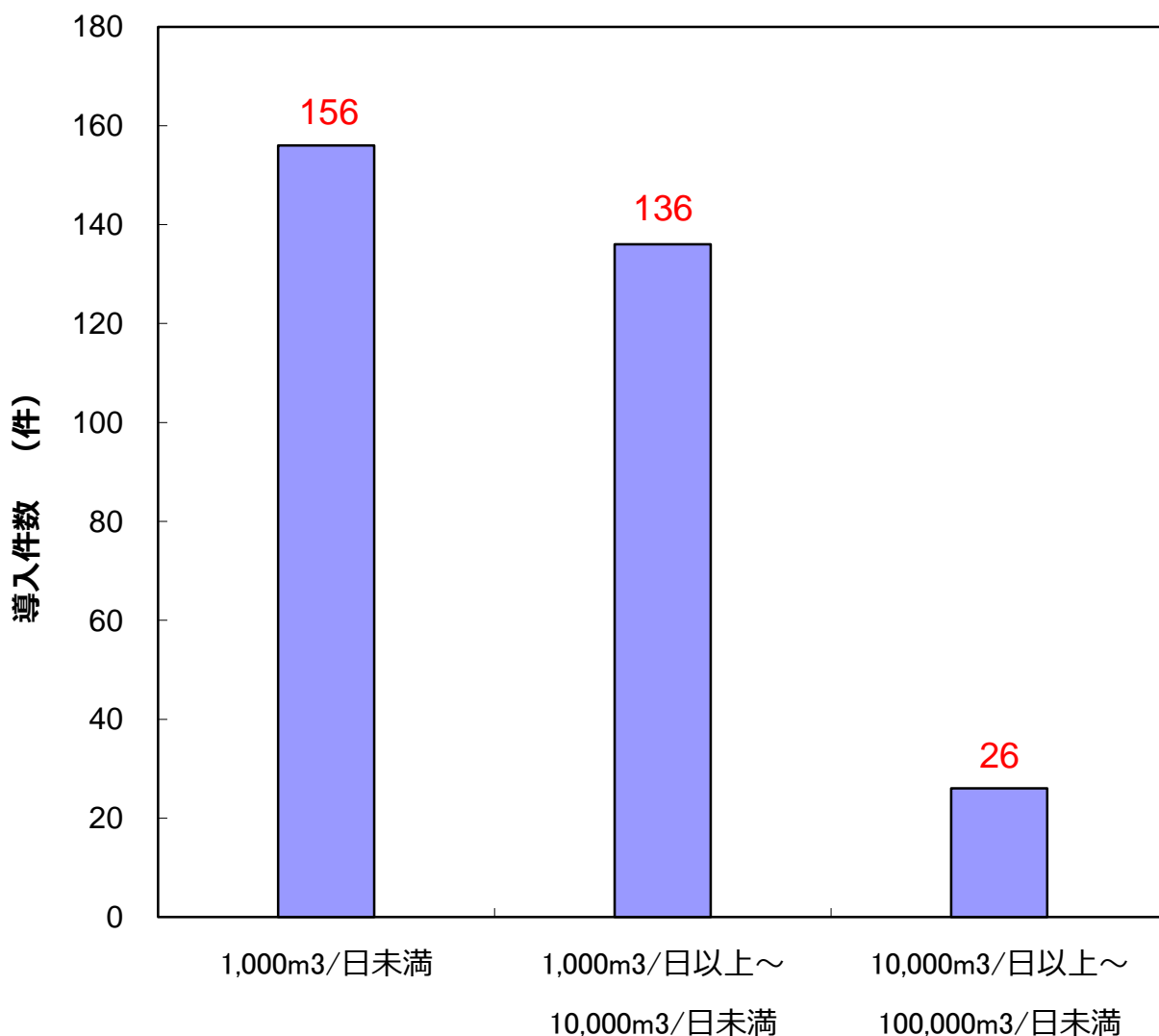
図2 浄水プロセスにおける処理水量別紫外線処理設備導入状況
