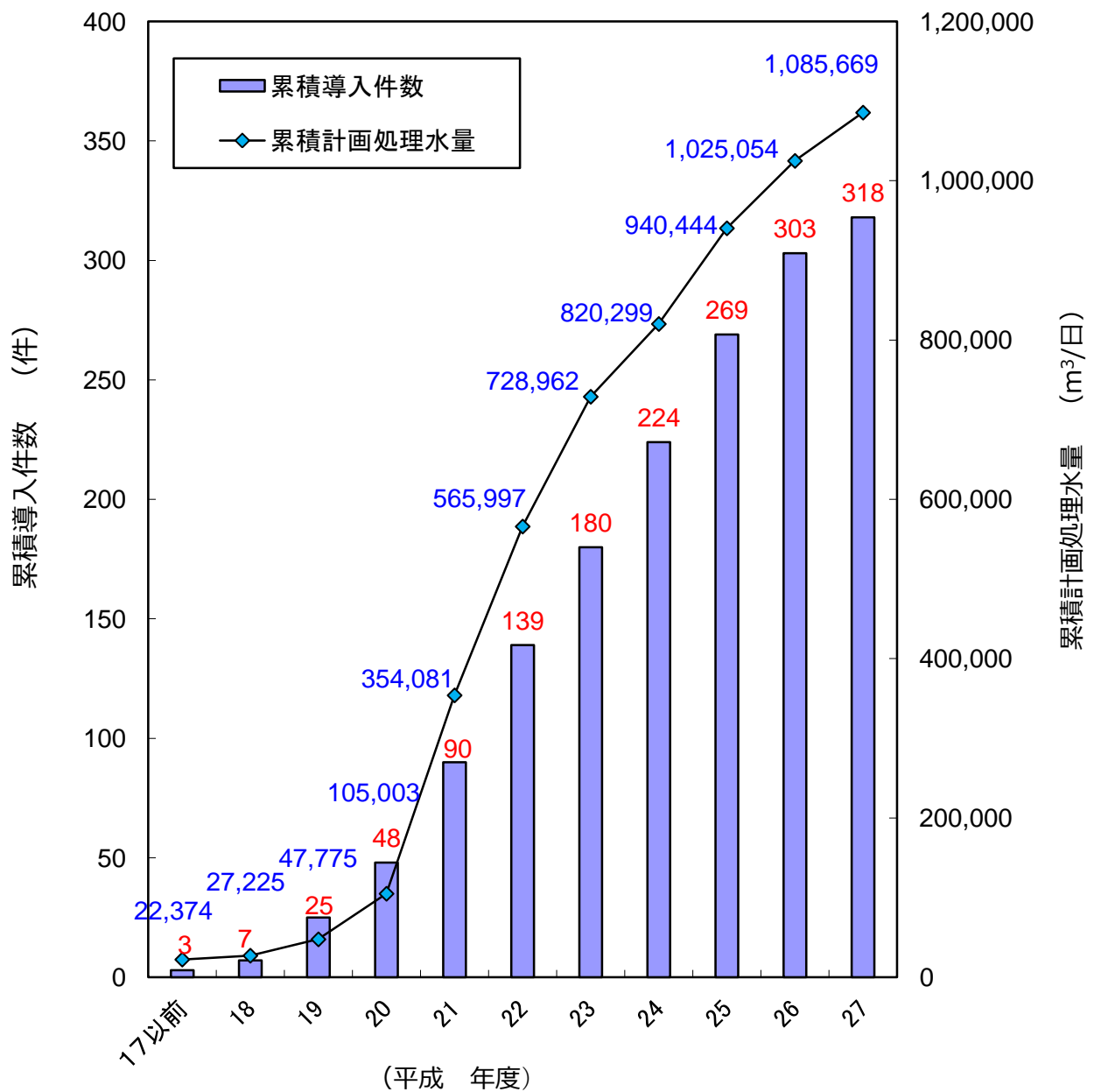
図1 浄水プロセスにおける紫外線処理設備の導入状況
