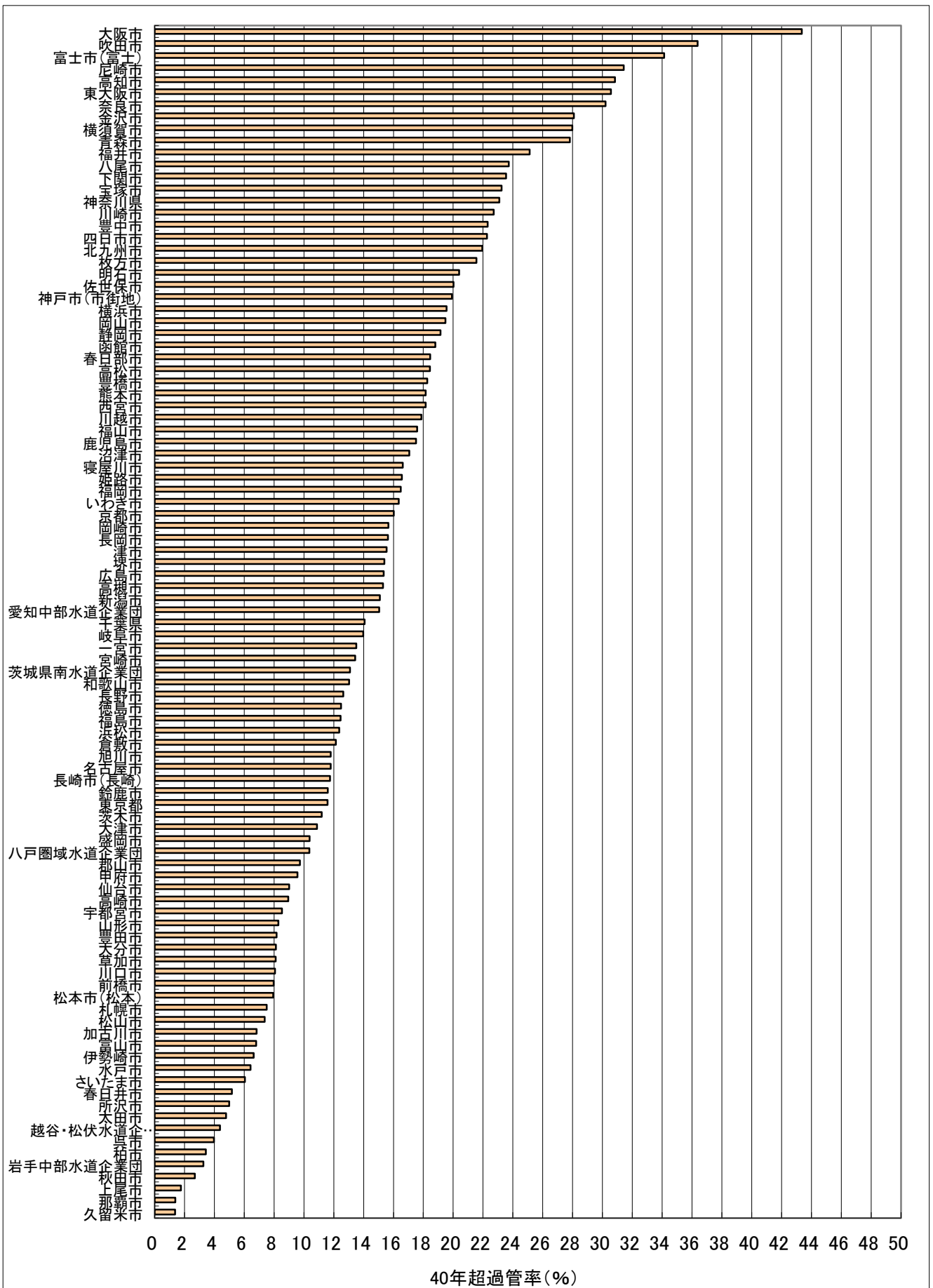
図 現在給水人口20万人以上の上水道99事業者における「40年超過管率」 (平成26年度)
