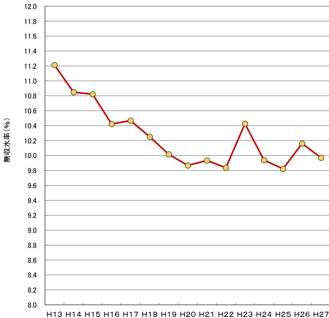
図1-3 日本の上水道事業における無収水率の推移(H13~H27、上水) JWRC
