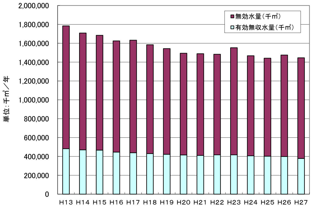
図1-1 日本の上水道事業における無収水量の年次別推移 -水道統計に基づく試算結果-
