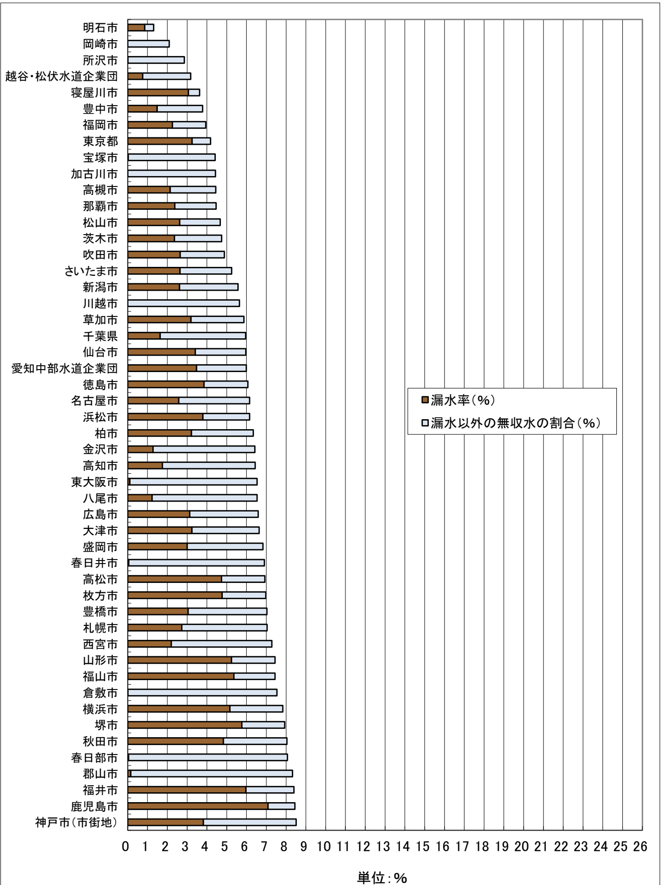
図2-1 平成27年度現在給水人口20万人以上の99上水道事業者の無収水率 (率の低い順) - その1 -
