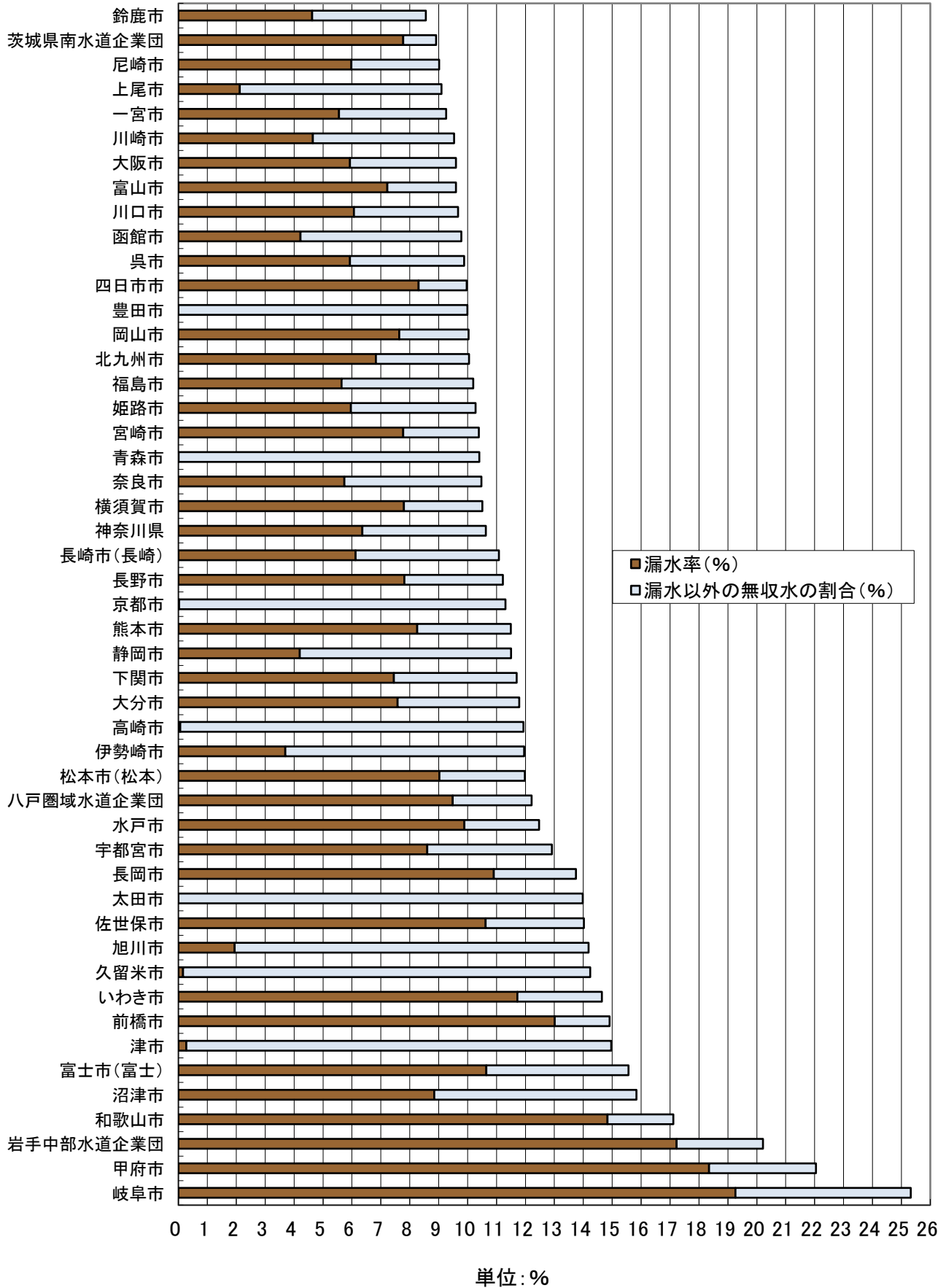
図2-2 平成27年度現在給水人口20万人以上の99上水道事業者の無収水率 (率の低い順) - その2 -
