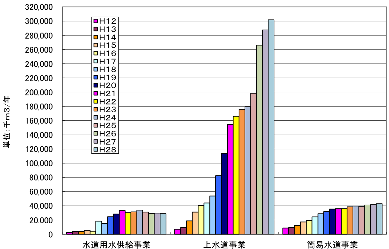
図2 膜ろ過浄水施設(MF・UF・NF・ROの合計)による年間実浄水量の推移(事業別) JWRC
