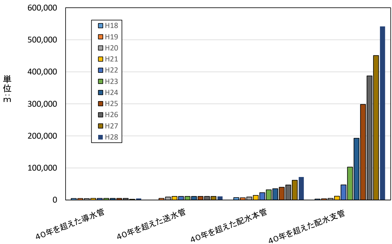
図8-2 40年を超えた水道管延長の推移 (札幌市)
