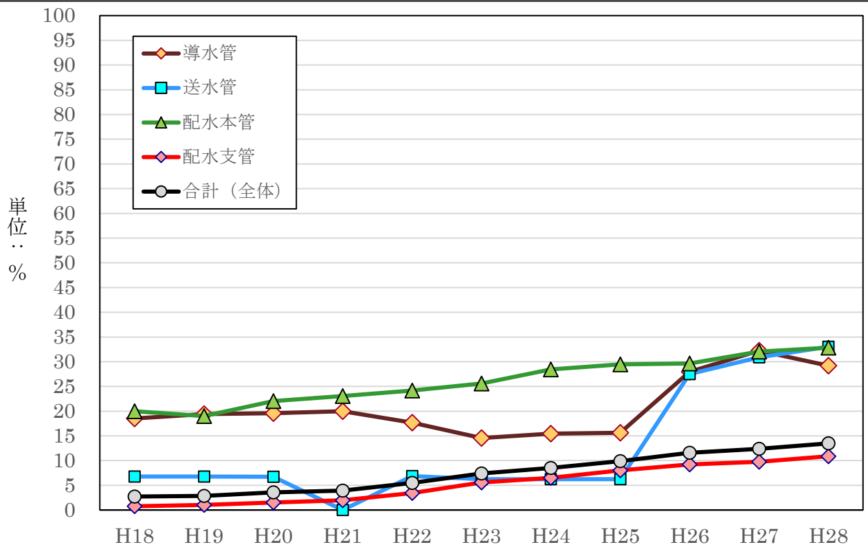
図2-1 40年超過管率の推移 (東京都)
