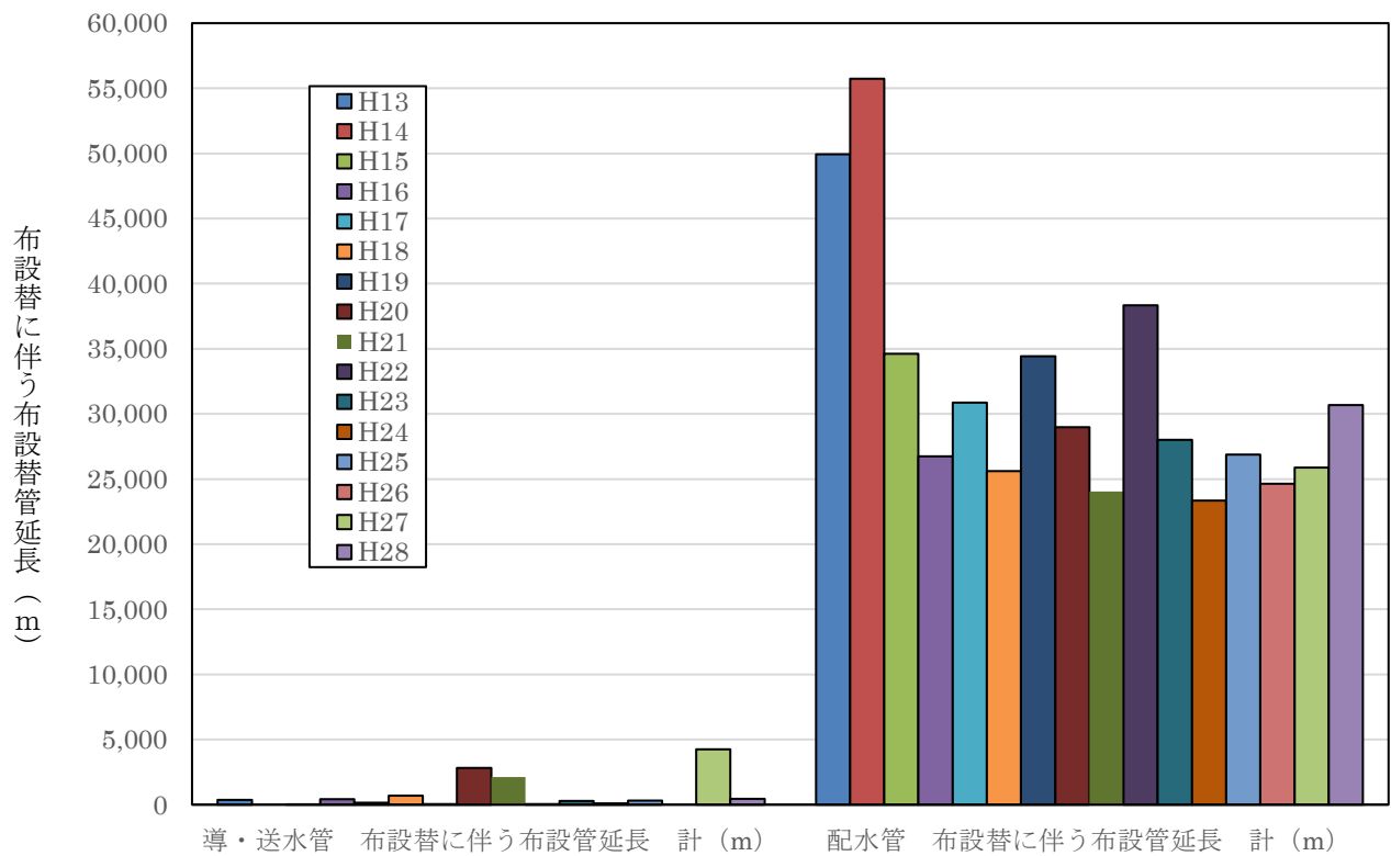
図2-9-2 導・送水管及び配水管別にみた布設替に伴う布設管延長の推移 (神戸市 (市街地))
