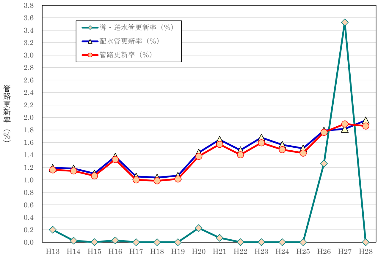
図2-10-1 導・送水管及び配水管別にみた管路更新率の推移 (川崎市)
