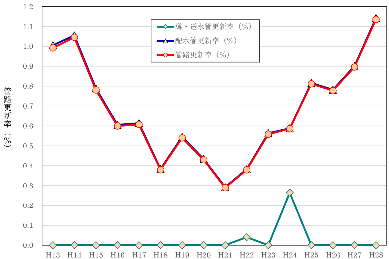
図2-8-1 導・送水管及び配水管別にみた管路更新率の推移 (京都市)
