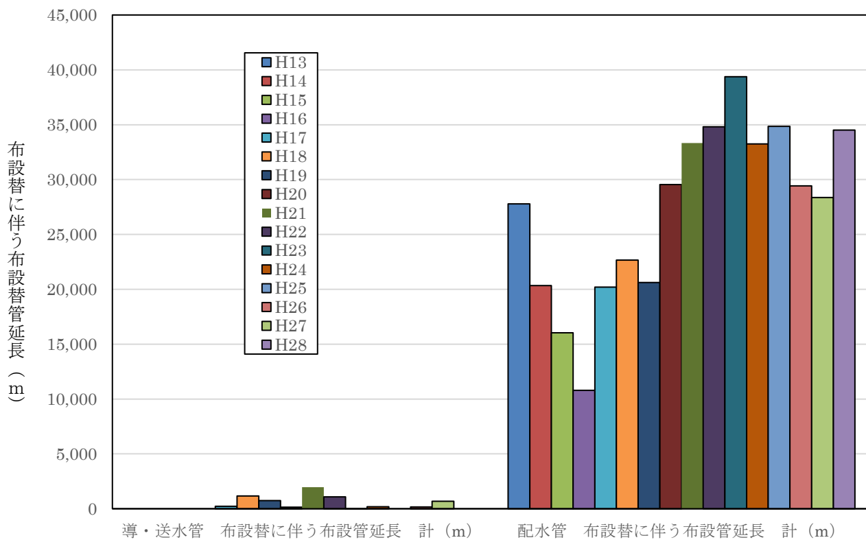
図2-11-2 導・送水管及び配水管別にみた布設替に伴う布設管延長の推移 (さいたま市)
