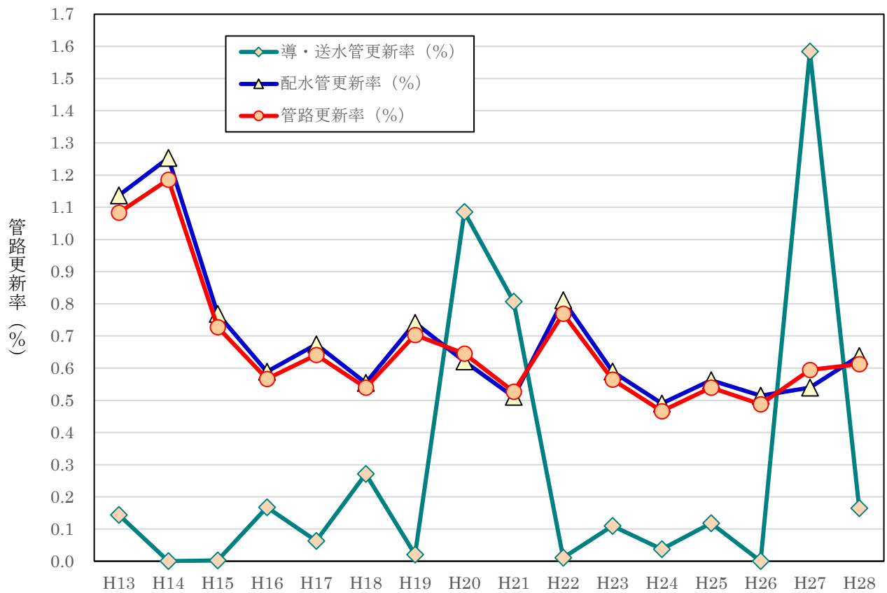
図2-9-1 導・送水管及び配水管別にみた管路更新率の推移 (神戸市 (市街地))
