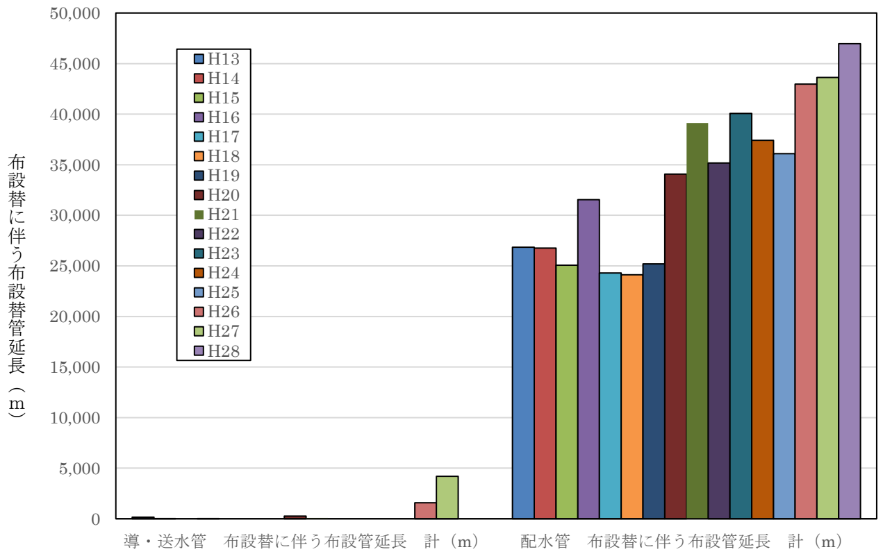
図2-10-2 導・送水管及び配水管別にみた布設替に伴う布設管延長の推移 (川崎市)
