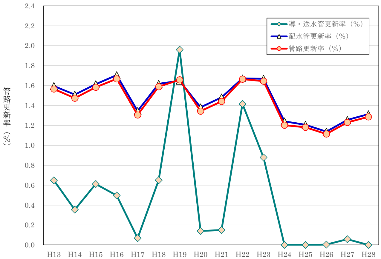
図2-6-1 導・送水管及び配水管別にみた管路更新率の推移 (名古屋市)
