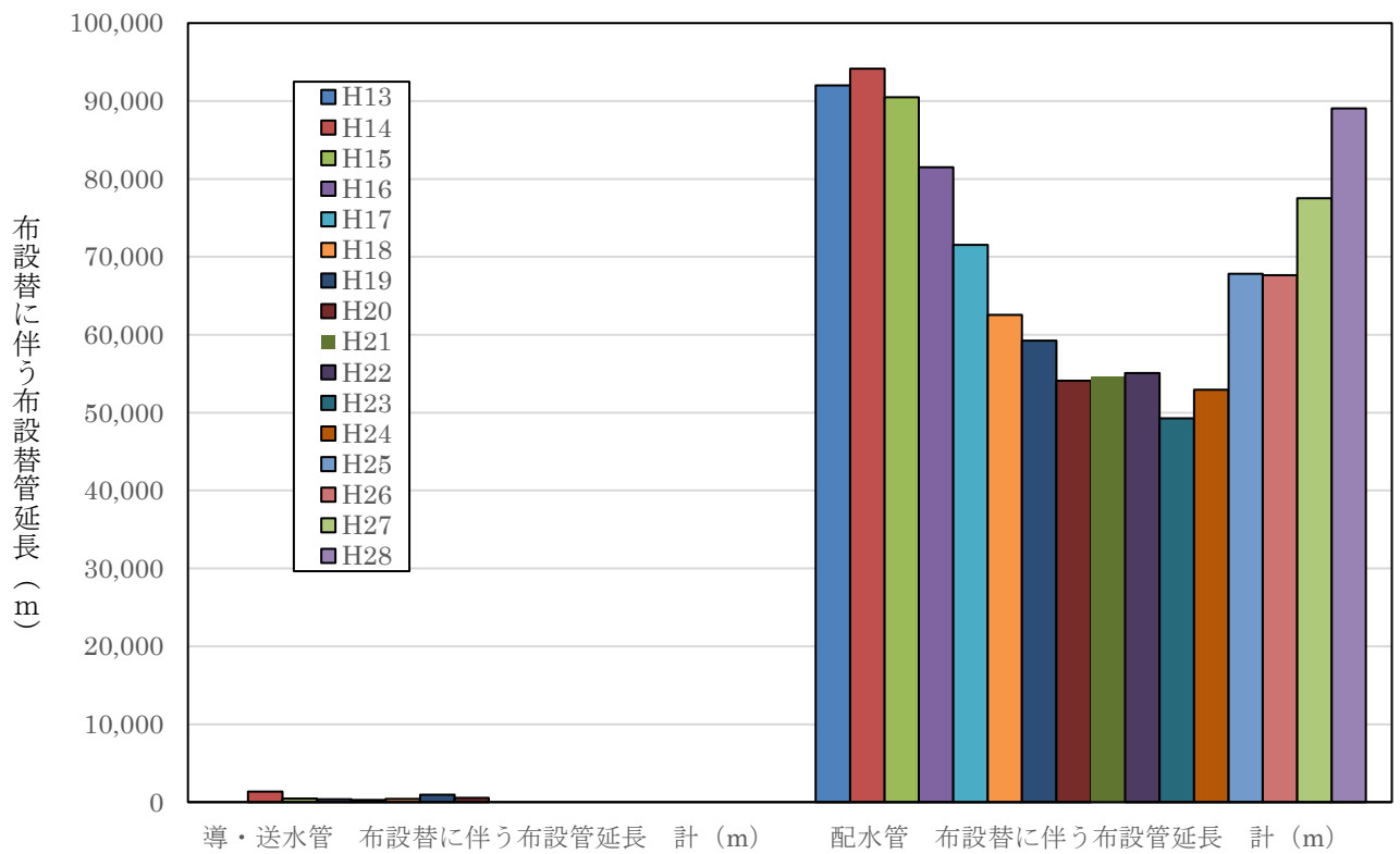
図2-7-2 導・送水管及び配水管別にみた布設替に伴う布設管延長の推移 (札幌市)
