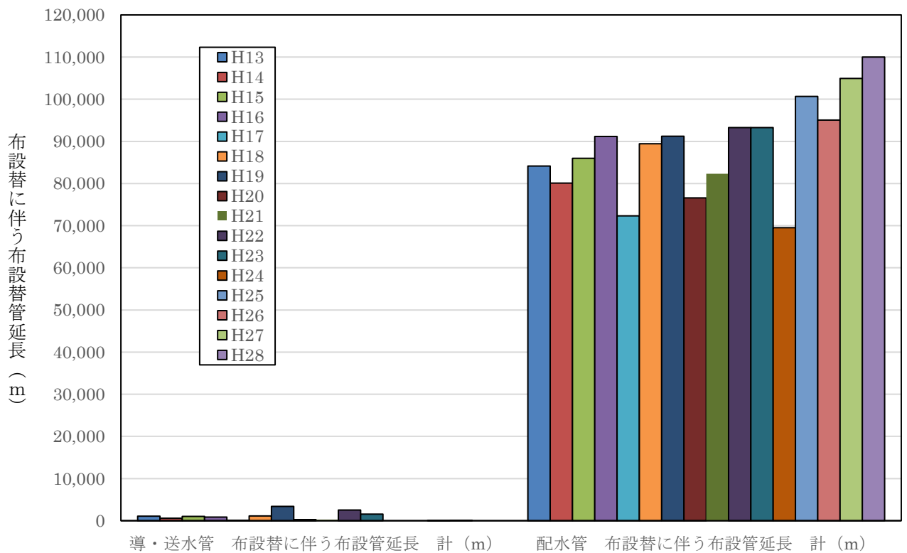
図2-6-2 導・送水管及び配水管別にみた布設替に伴う布設管延長の推移 (名古屋市)
