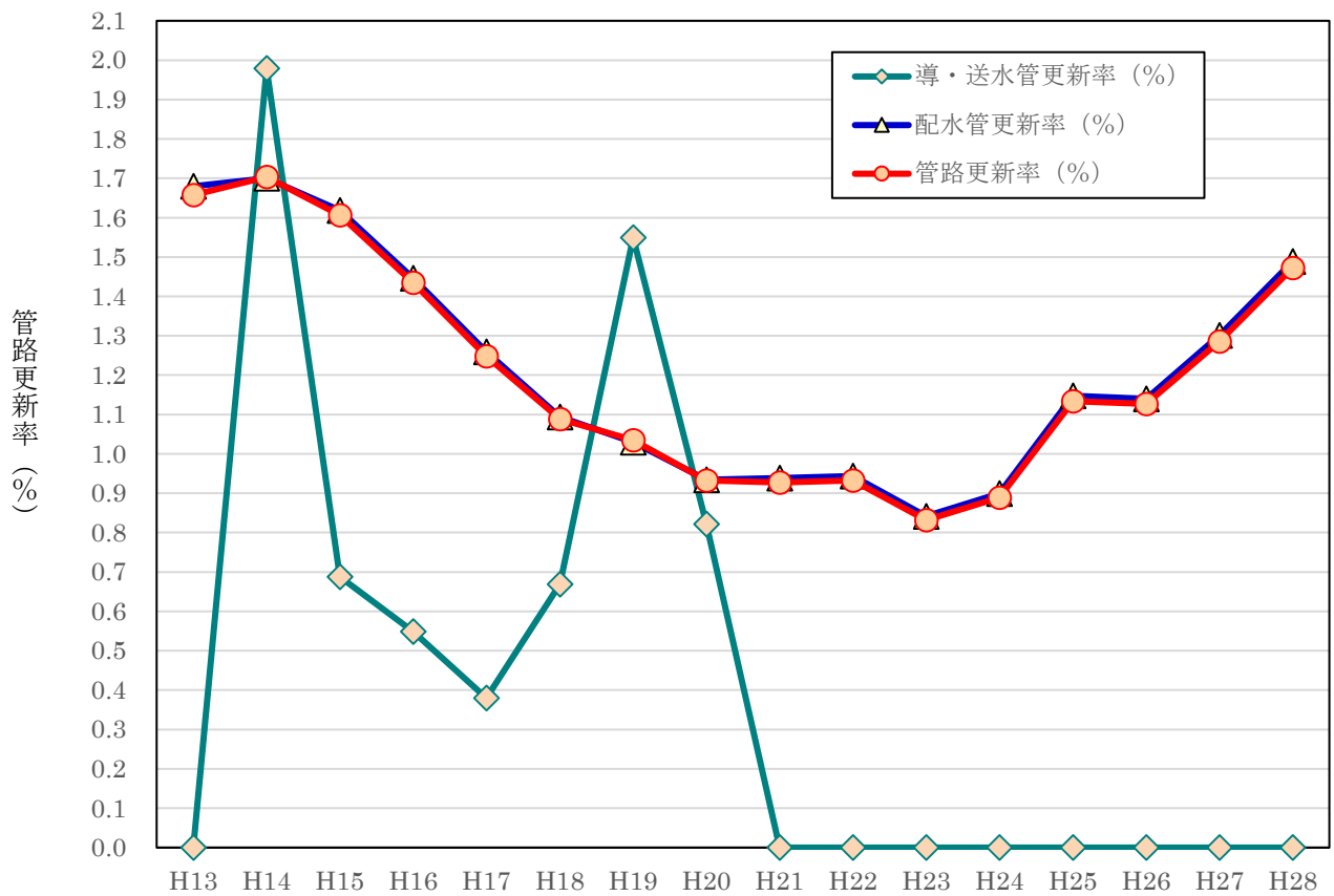
図2-7-1 導・送水管及び配水管別にみた管路更新率の推移 (札幌市)
