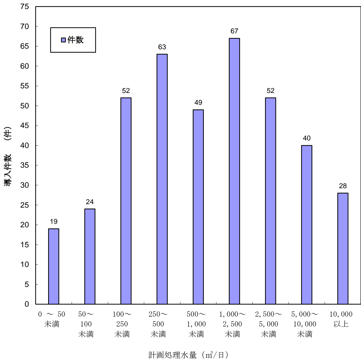
図2 浄水プロセスにおける処理水量別紫外線処理設備導入状況 (平成 30 年度)
