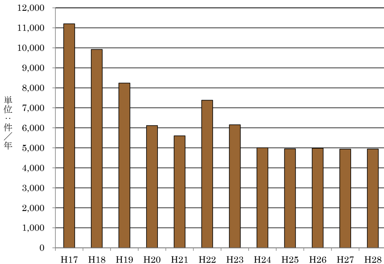
図2 幹線管路の事故発生件数の推移 (全国、用供+上水)
