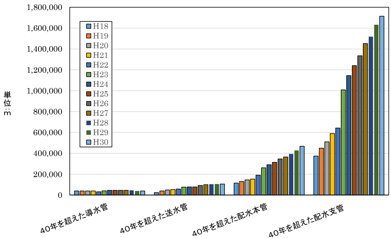
図6-2 40年を超えた水道管延長の推移 (横浜市)
