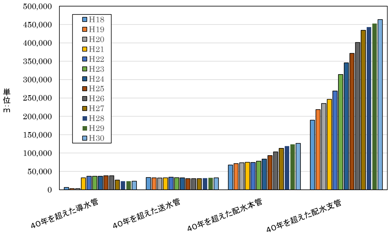
図12-2 40年を超えた水道管延長の推移 (川崎市)
