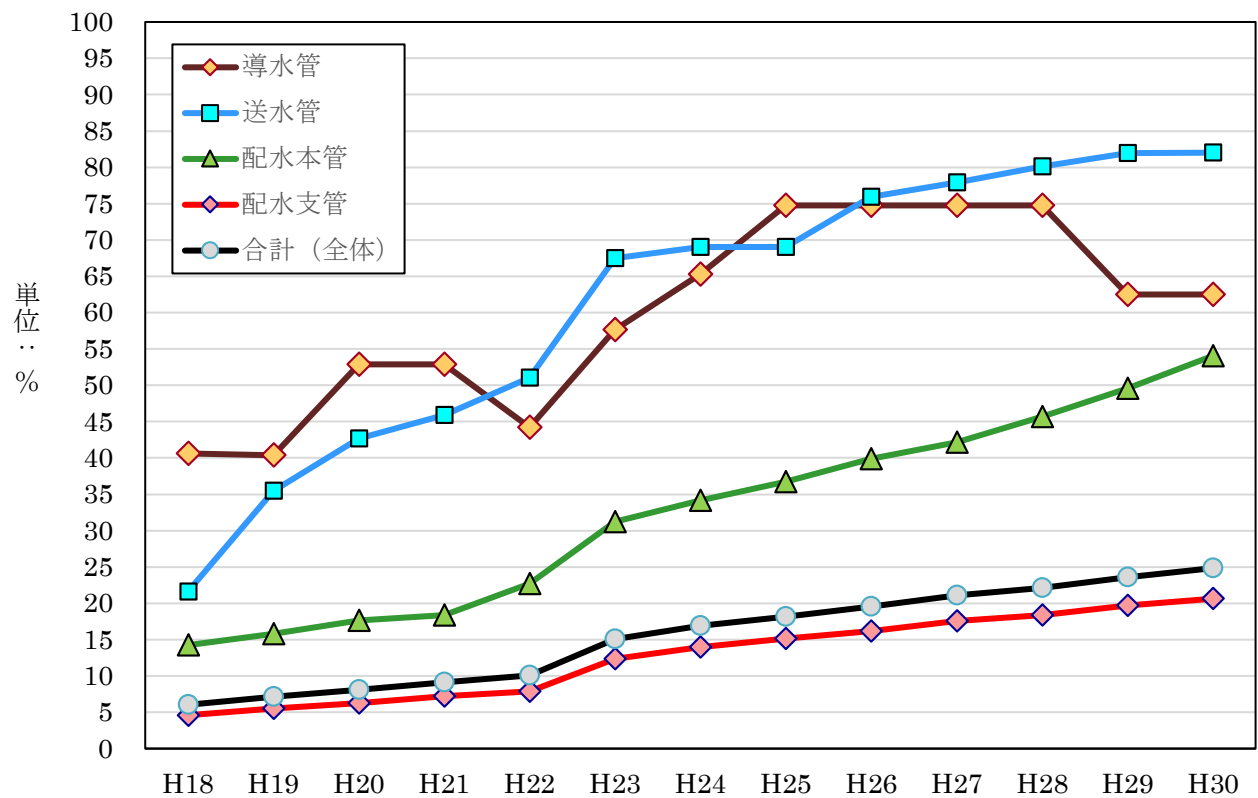
図6-1 40年超過管率の推移 (横浜市)
