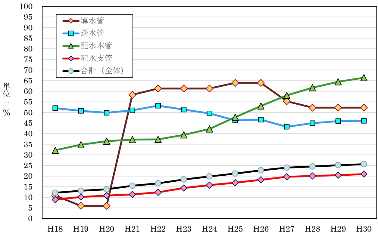
図12-1 40年超過管率の推移 (川崎市)
