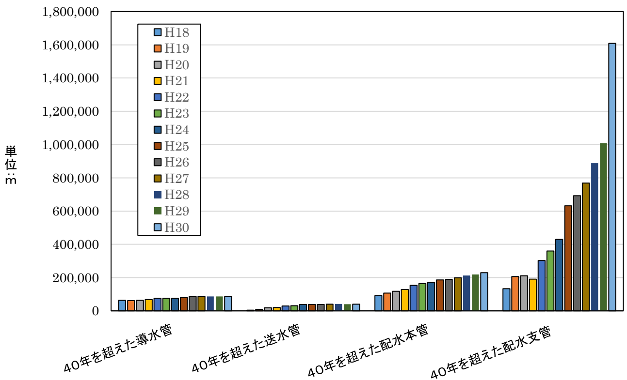
図5-2 40年を超えた水道管延長の推移 (名古屋市)
