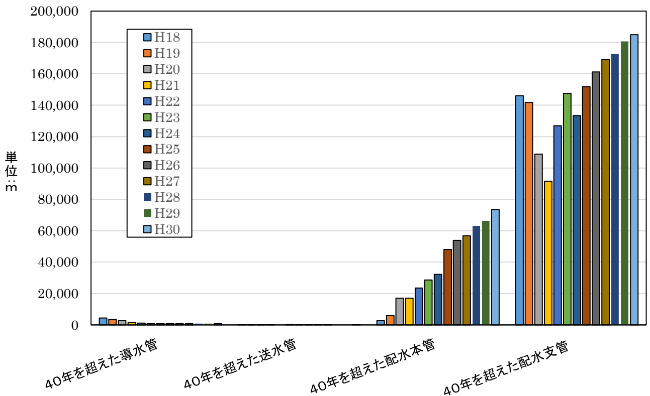
図10-2 40年を超えた水道管延長の推移(さいたま市)
