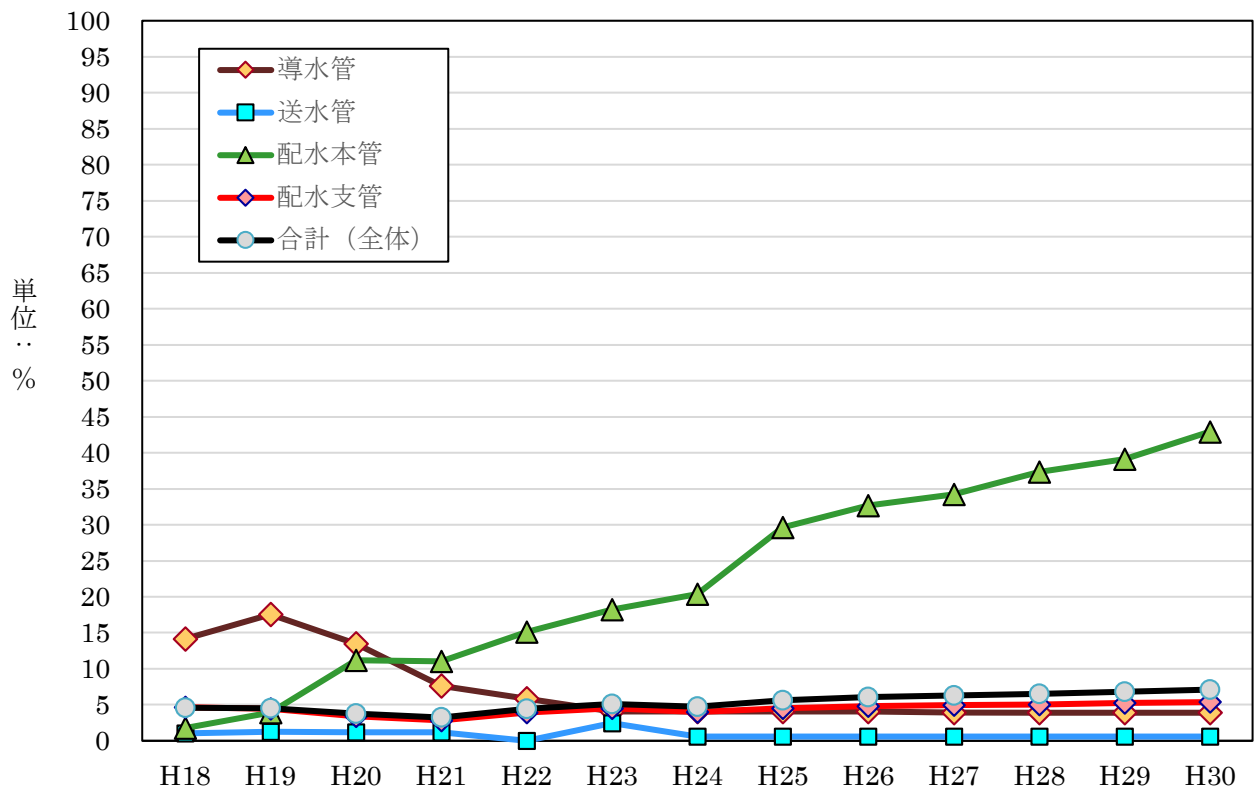
図10-1 40年超過管率の推移 (さいたま市)
