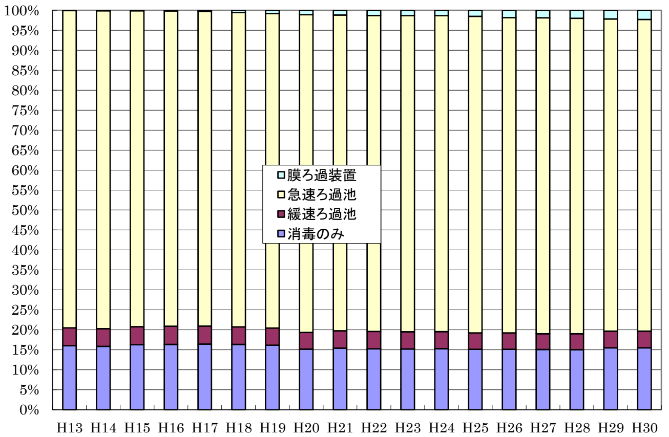
図2-2 浄水方法別計画浄水量の推移(用供+上水)ー構成割合ー
