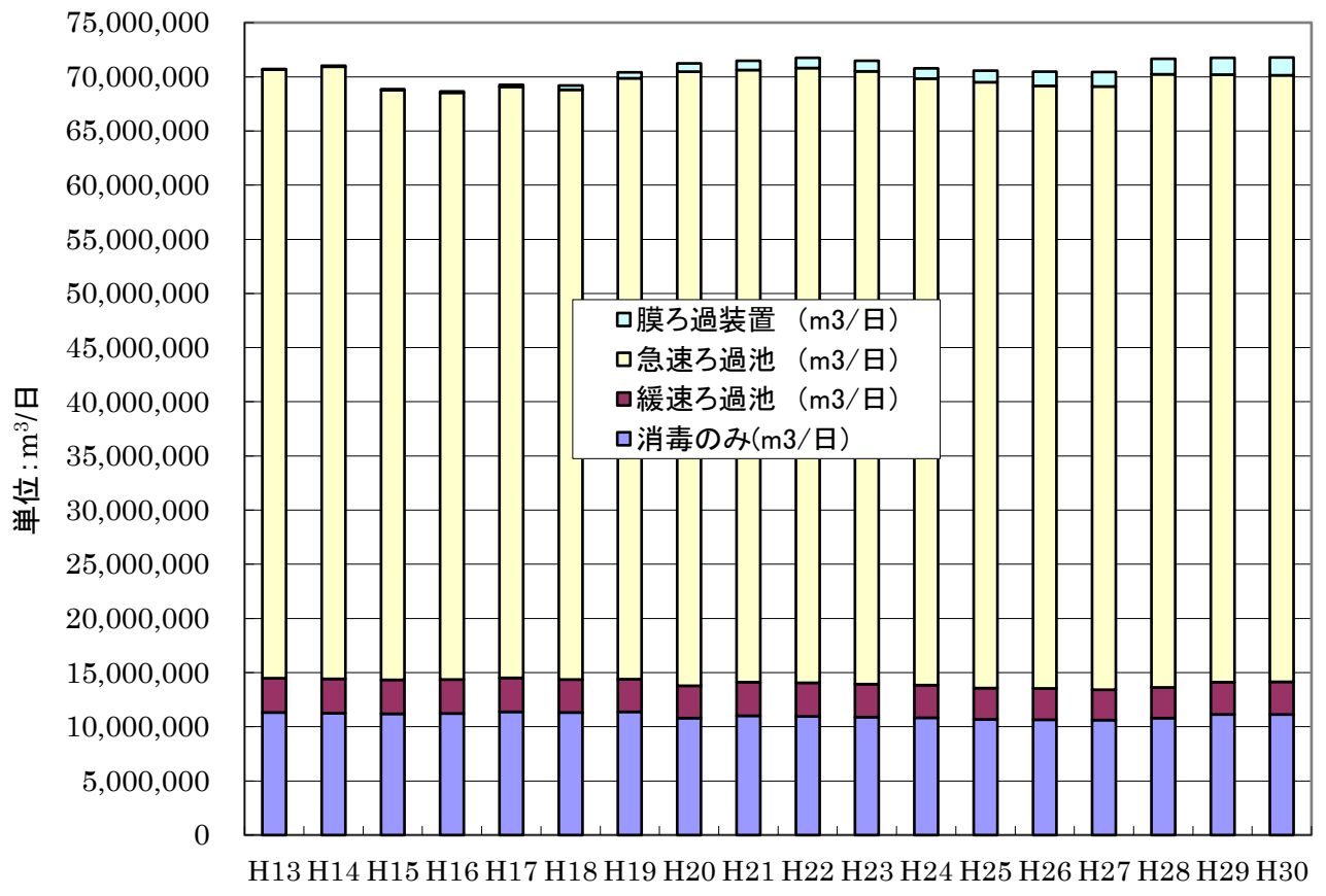
図2-1 浄水方法別計画浄水量の推移(用供+上水)ー積み上げー
