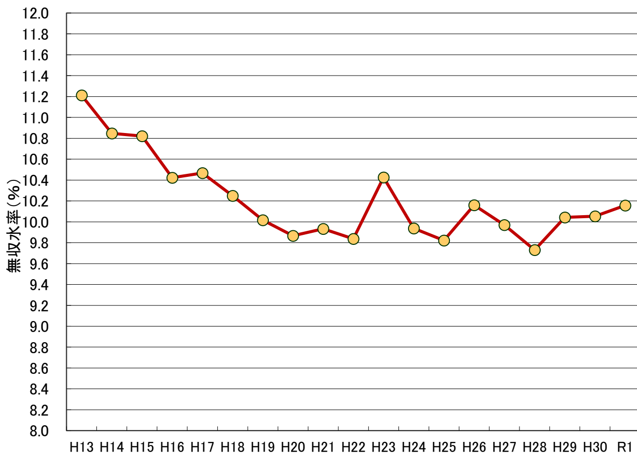
図1-3 日本の上水道事業における無収水率の推移(H13~R1、上水)
