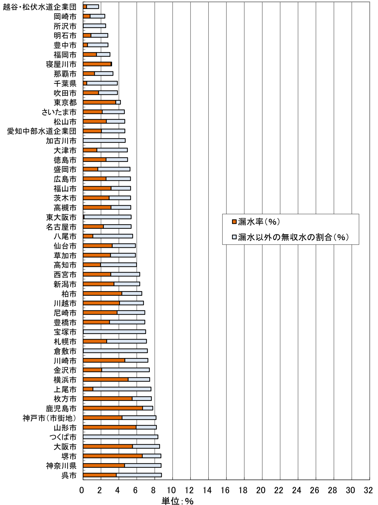
図2-1 現在給水人口20万人以上の上水道100事業者の無収水率 (令和元年度、無収水率の低い順)
