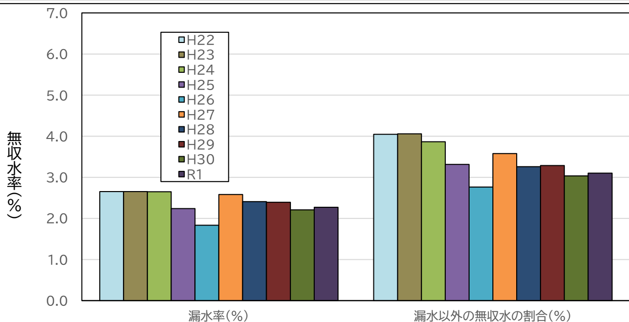
図6-2 無収水率及びその内訳の推移(要因別)(名古屋市上下水道局)
