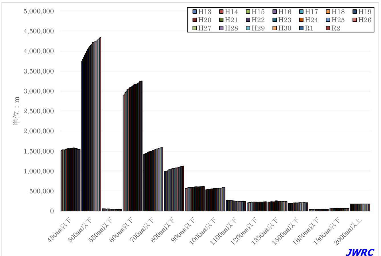
図 1 - 3 : 上水道事業における配水管延長の推移その 2 (全国、口径別)
