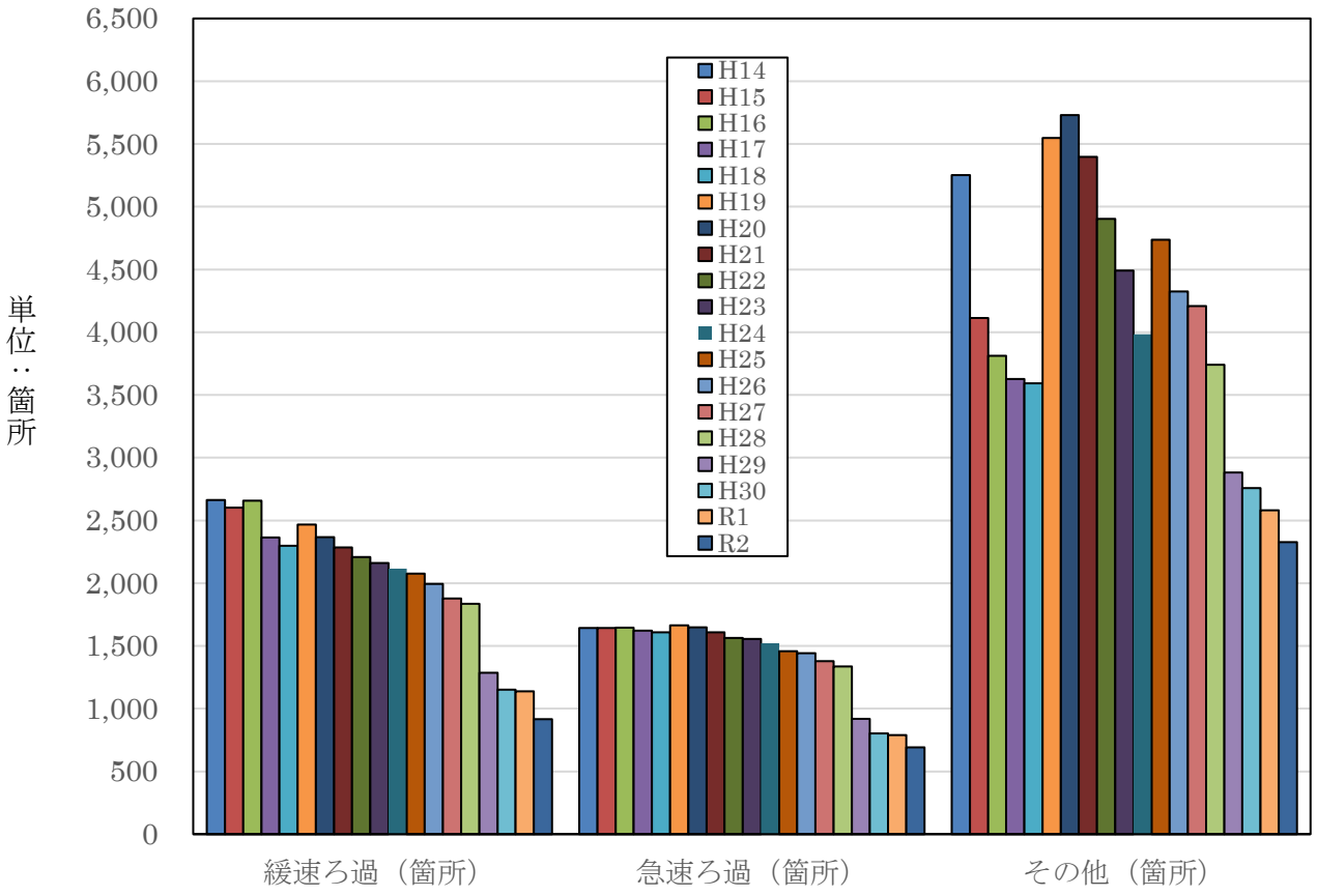
図1-2 簡易水道事業における浄水施設数の推移 (浄水方法別)
