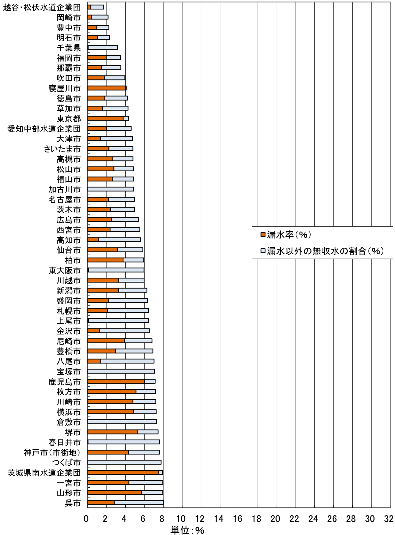
図2-1 現在給水人口20万人以上の上水道100事業者の無収水率 (令和2年度、無収水率の低い順)
