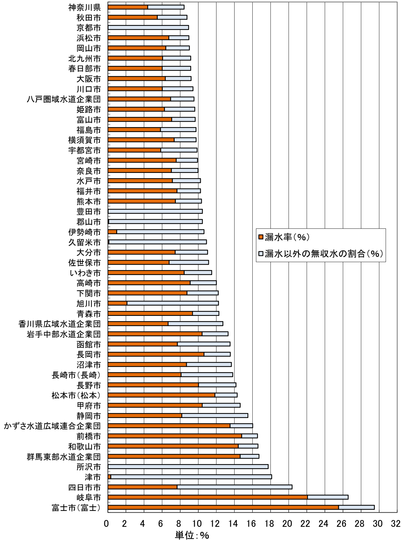
図2-2 現在給水人口20万人以上の上水道事100業体の無収水率 (令和2年度、無収水率の低い順)
