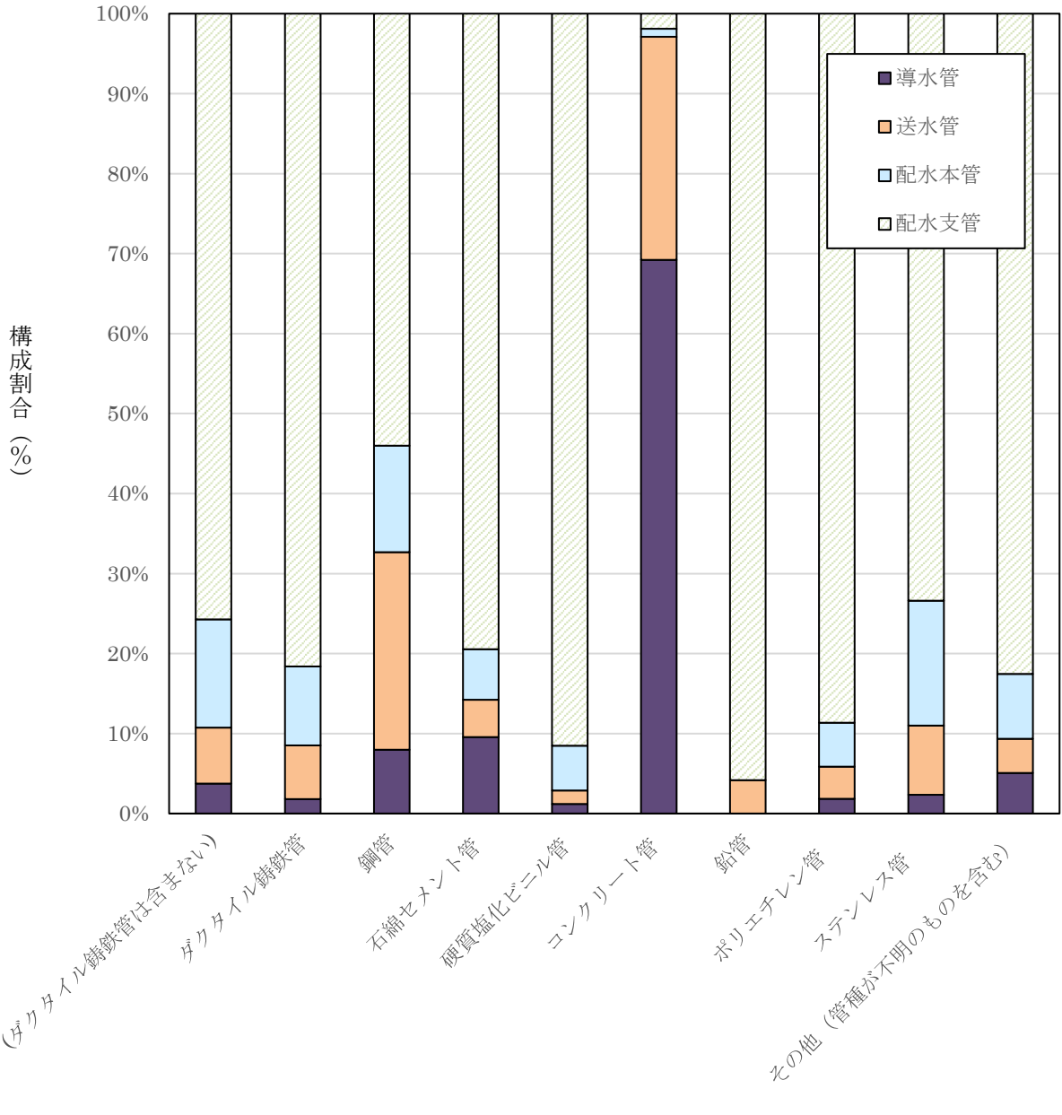
図 2-1 管種別にみた 導水管・送水管・配水本管・配水支管の延長 (構成割合) (令和3年度、全国、用供+上水)
