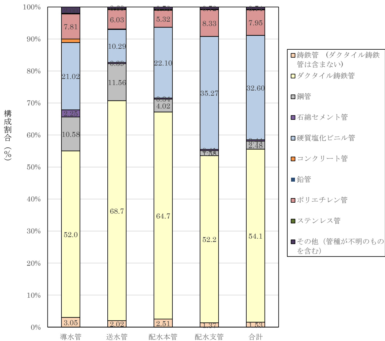
図 1 - 2 導水管・送水管・配水本管・配水支管別にみた 管種別延長の構成割合 (令和3年度、全国、用供+上水)
