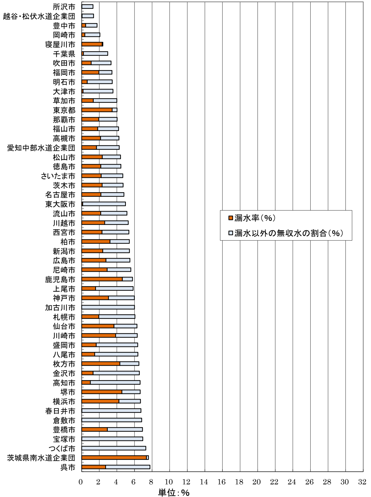
図2-1 現在給水人口20万人以上の上水道101事業者の無収水率 (令和3年度、無収水率の低い順)
