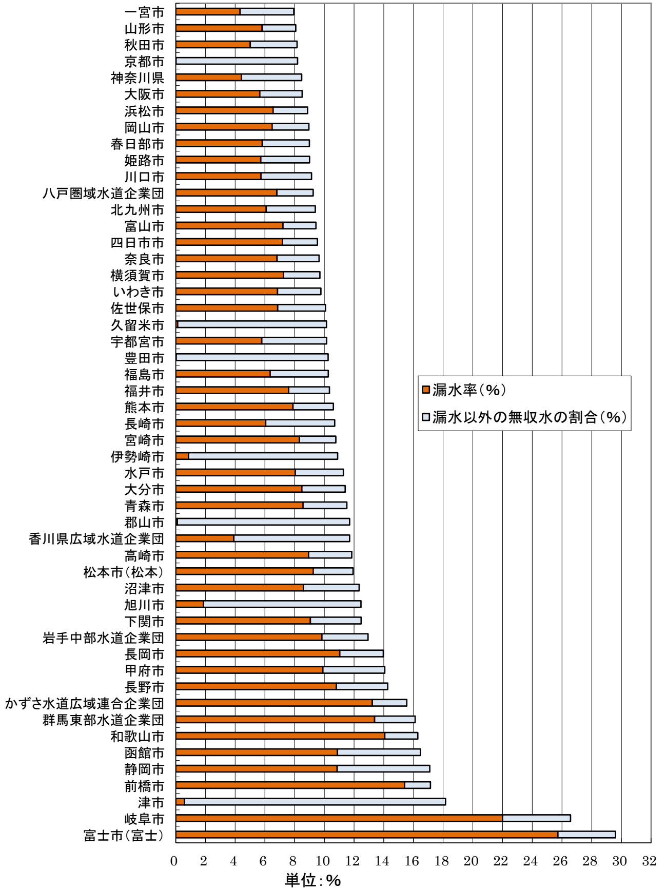
図2-2 現在給水人口20万人以上の上水道事101業体の無収水率 (令和3年度、無収水率の低い順)
